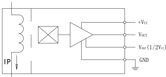
外部参考电路及接线图
