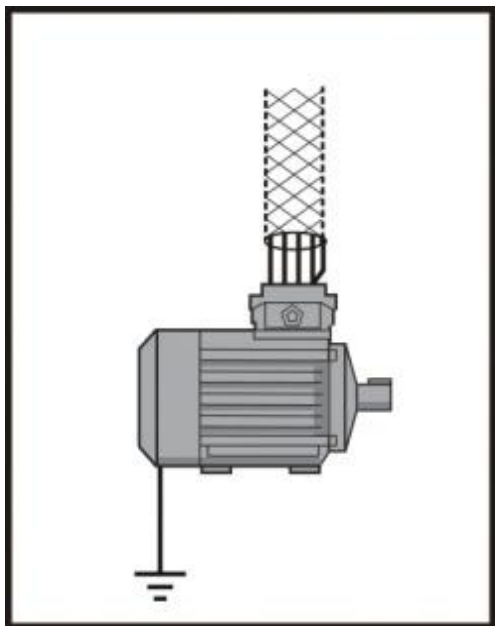
图 3-51 电机电缆屏蔽接地
