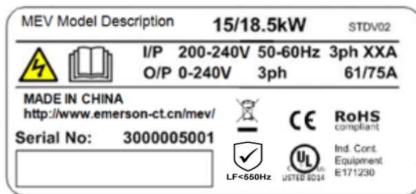
图 A-3 变频器铭牌
