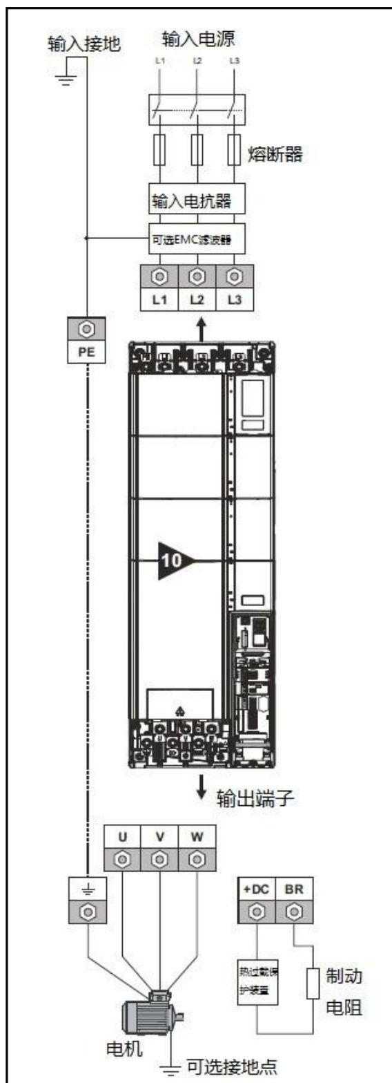
图 3-30 Size 9E、10 主回路输入输出连接图
