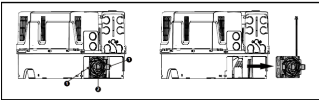
图 3-21 风扇拆除示意图
