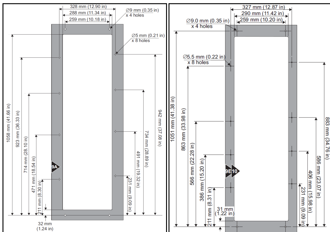
图 3-15 Size 9A (左)、Size 9E&10 (右) 透壁式安装尺寸图
