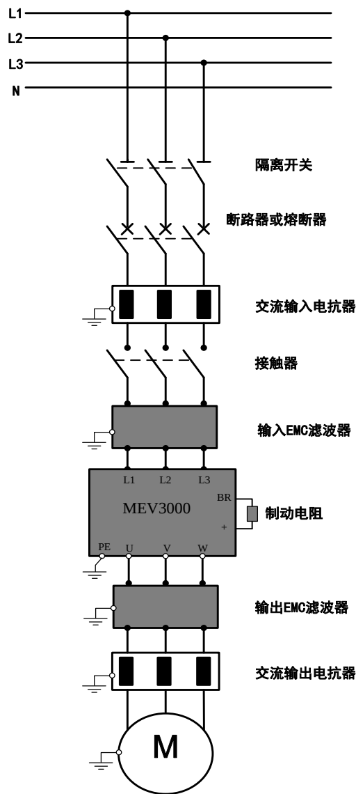
图 3-23 变频器与选配件的连接
