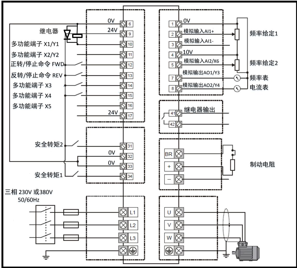
图3-32 端子连接图
