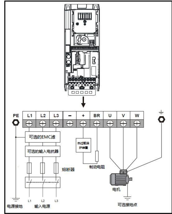
图 3-25 Size3 主回路输入输出连接图
