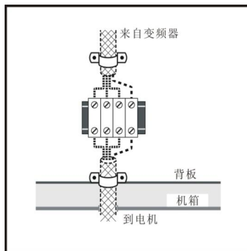
图 3-54 将电机线缆连至柜内接线端子
