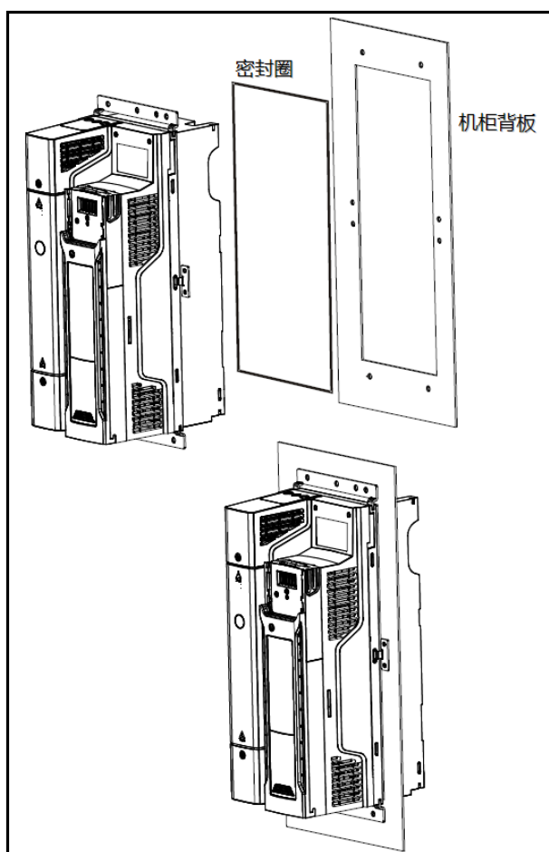
图 3-18 安装密封圈
