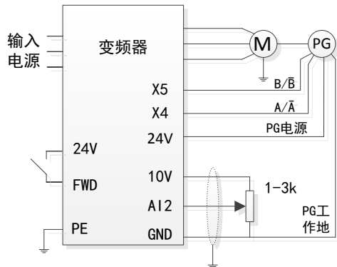
图 5-23 PG 速度闭环控制系统接线图
