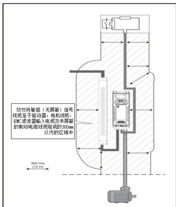
图 3-46 变频器线缆间隔
