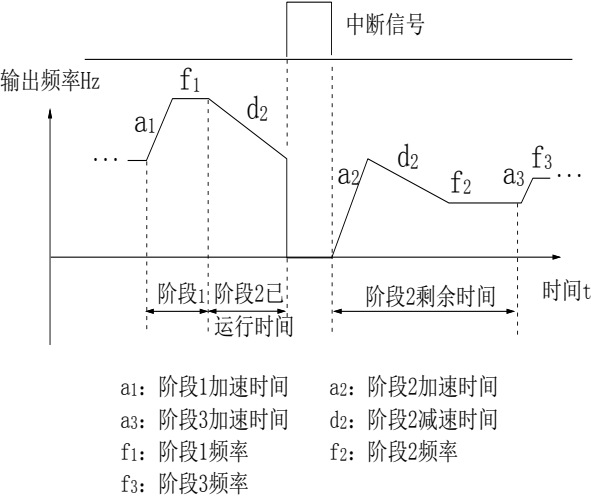
图 5-59 PLC 起动方式 2
