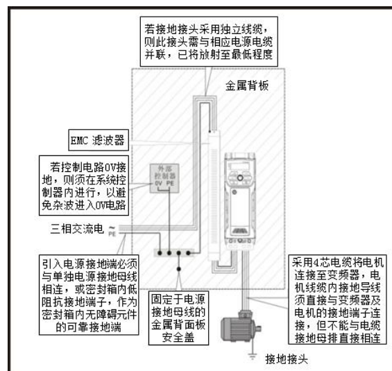
图 3-45 一般 EMC 机壳所示接地连接
