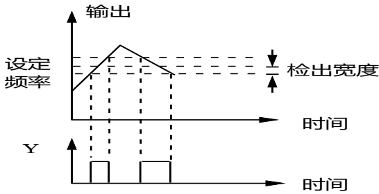
图 5-42 频率到达信号输出示意图
