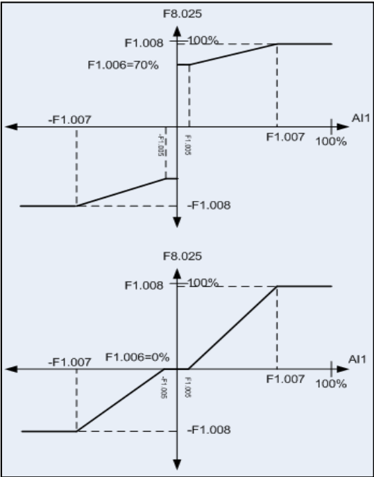
图 5-6 模拟输入 AI1 给定正作用特性
