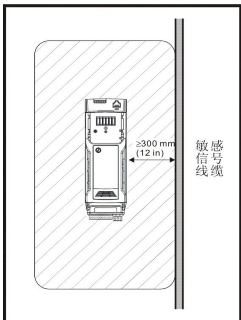
图 3-49 敏感信号电路间距
