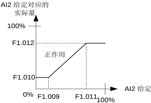
图 5-8 模拟输入 AI2 给定正作用特性
