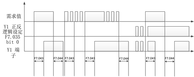
图5-45 输出开通/关闭延时
