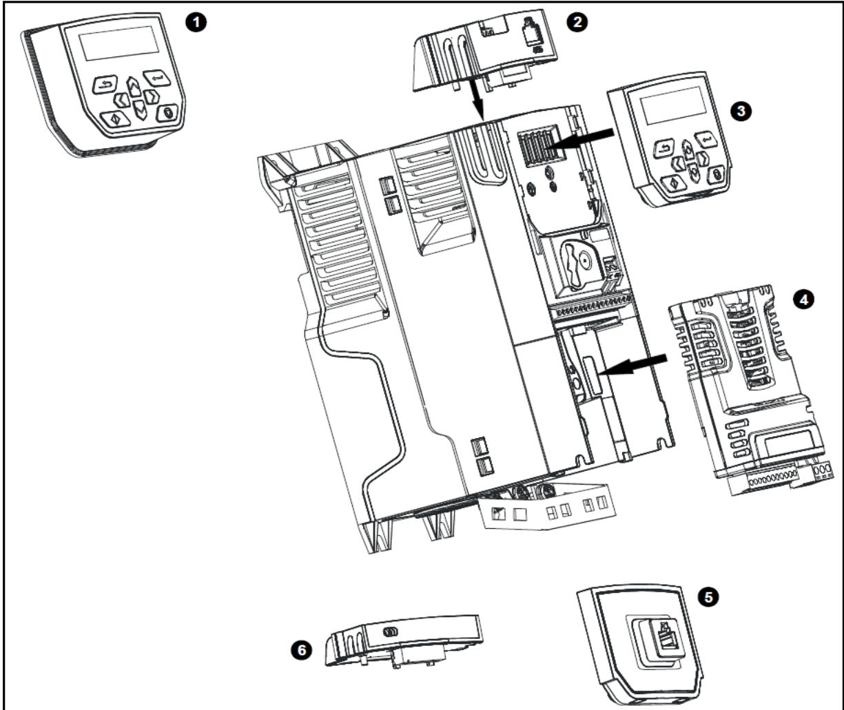
图 2-5 MEV3000 可支持的配件
