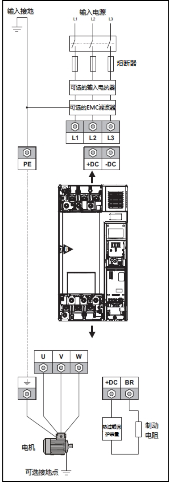
图 3-29 Size7~9A 主回路输入输出连接图
