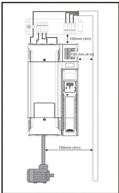
图 3-48 电源及接地线缆间距 (Size7~11)
