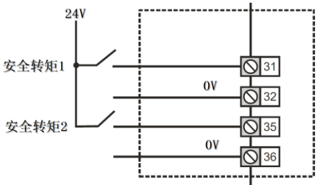
图 3-33 Frame 5-11 STO 端子连接图
