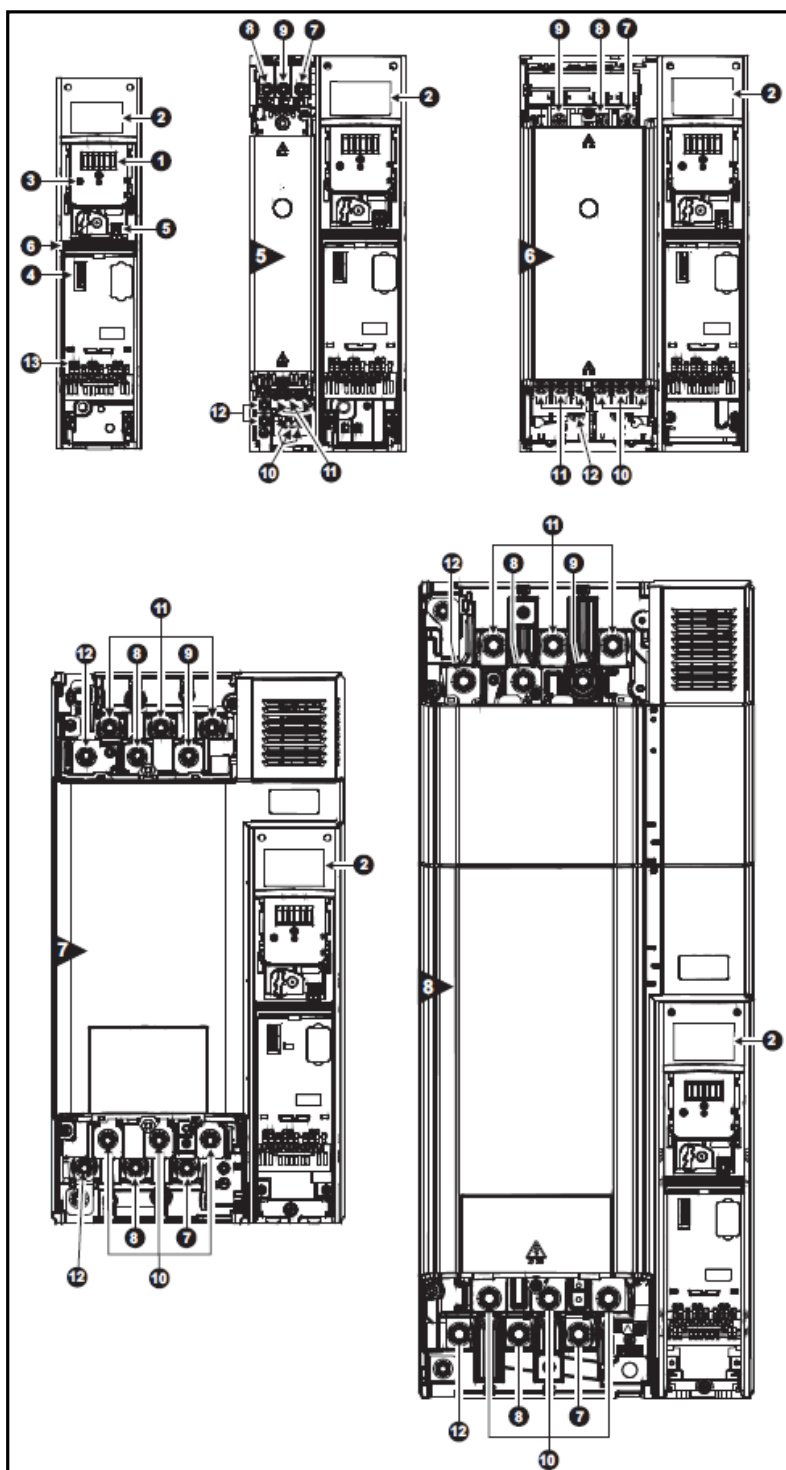
图 2-2 Size 5~8(11kW - 75kW)变频器各部位名称示意图
