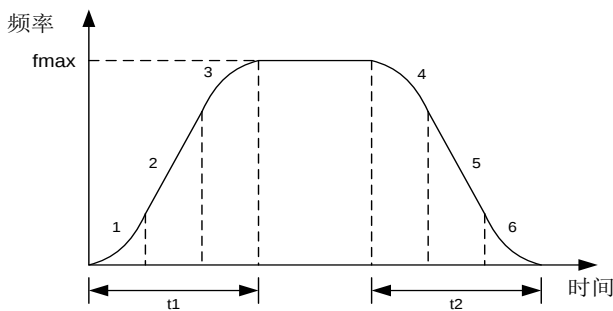
图 5-12 S 曲线加减速
