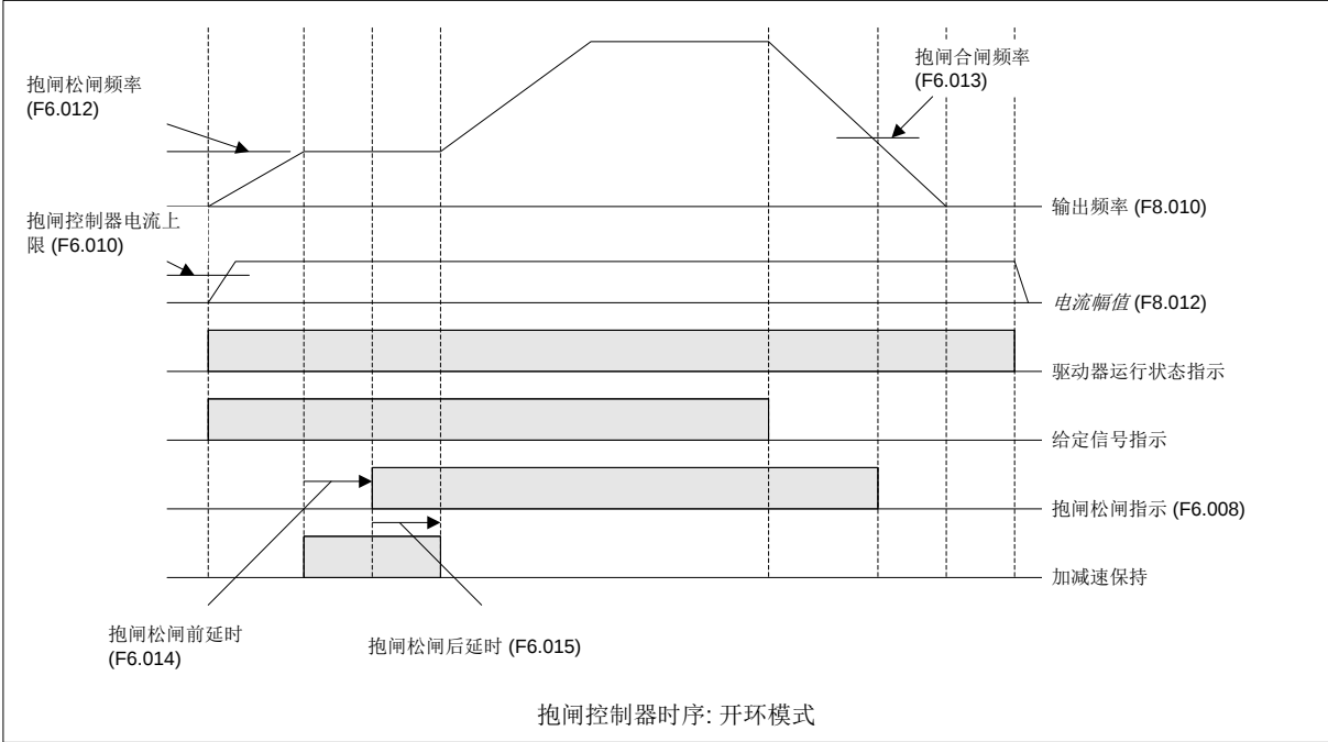
图 5-32 抱闸控制器时序：开环模式
