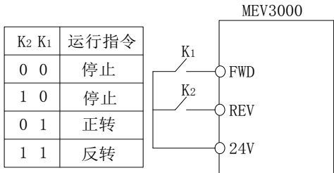
图 5-39 两线式运转模式 2
