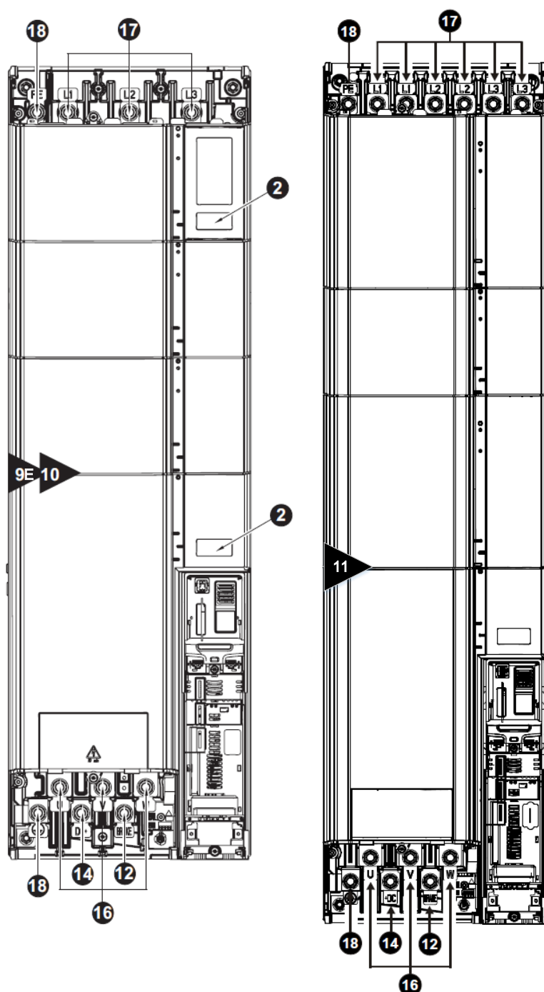
图 2-4 Size 9E(90~110kW)、Size 10~11(132kW - 250kW)变频器各部位名称示意图
