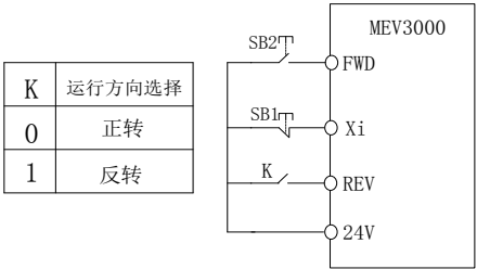
图 5-41 三线式运转模式 2
