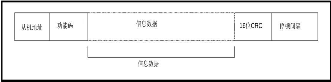
附图 8 帧格式
