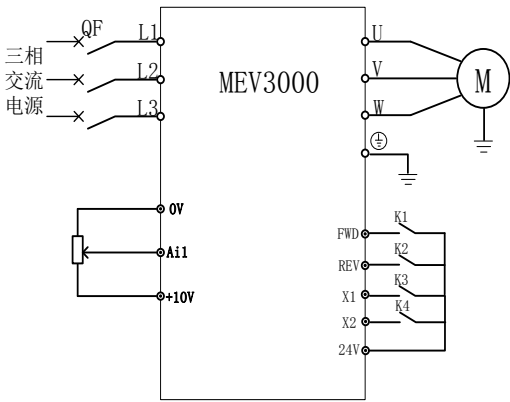
图 5-48 两线控制硬件接线图
