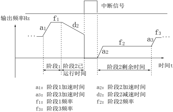
图 5-58 PLC 起动方式 1
