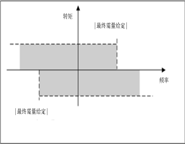
图 5-21 带频率限幅的双向转矩控制
