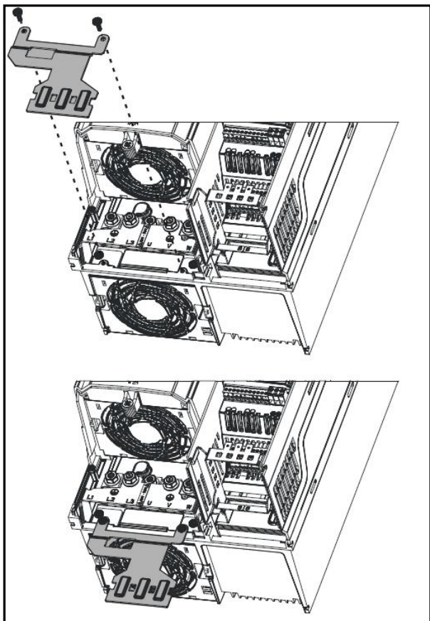
图 3-38 Size6 接地夹钳安装示意图
