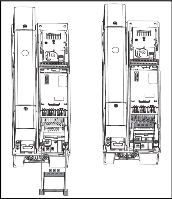
图 3-36 Size5-8 接地支架安装示意图（size5 为例）
