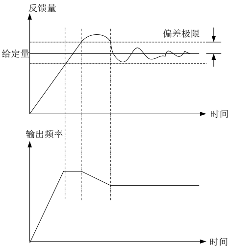
图 5-28 偏差极限示意图 1
