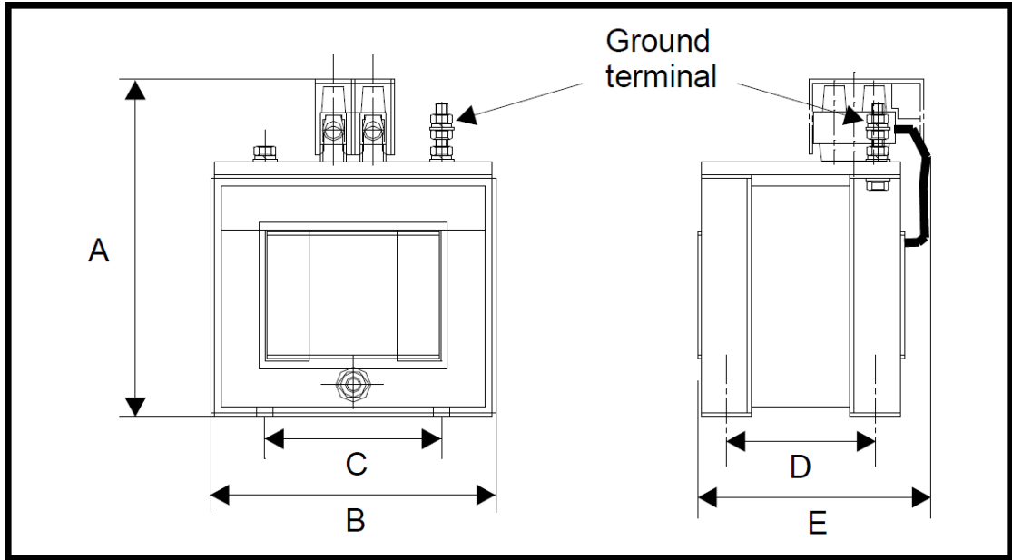
附图 1 交流输入电抗器外形图（4402-0224，4402-0225，4402-0226）
