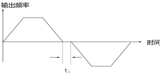
图 5-13 正反转死区时间
