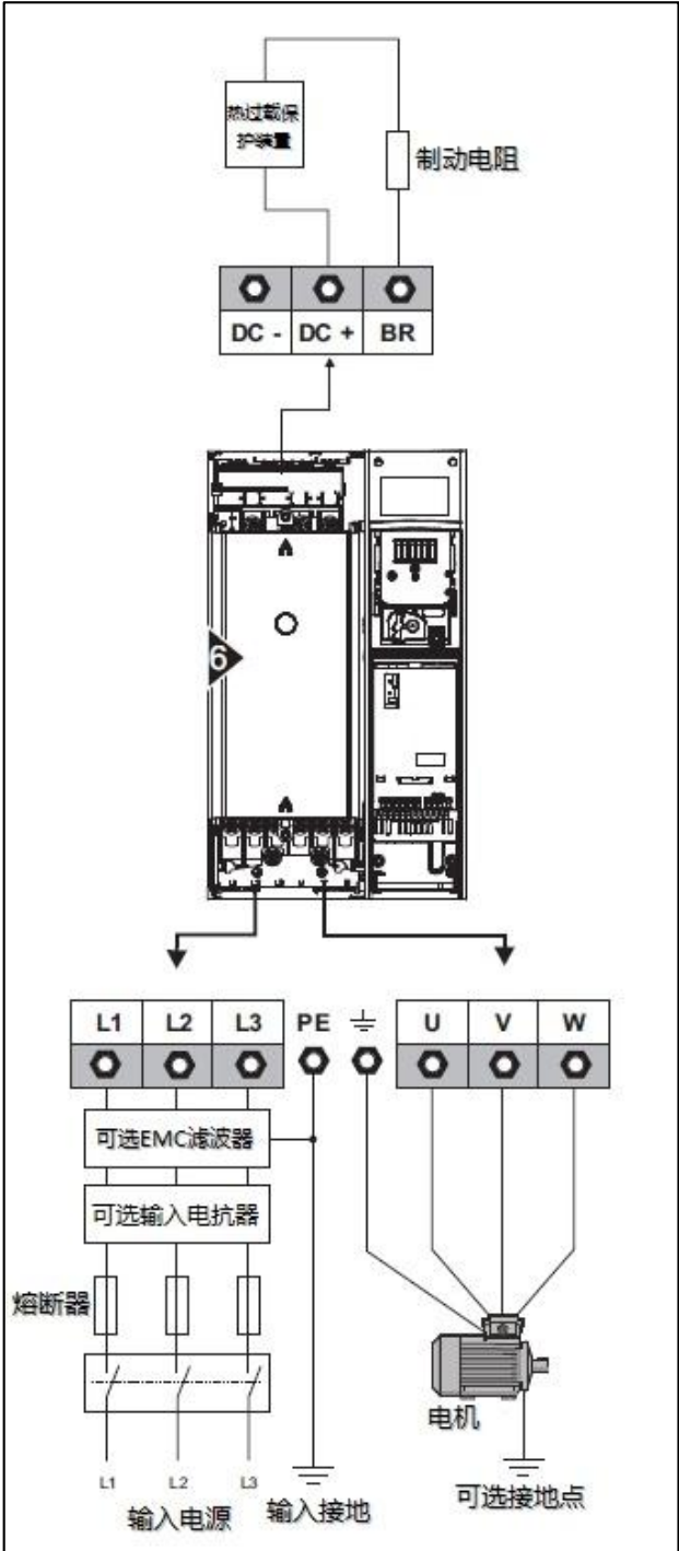
图 3-28 Size6 主回路输入输出连接图
