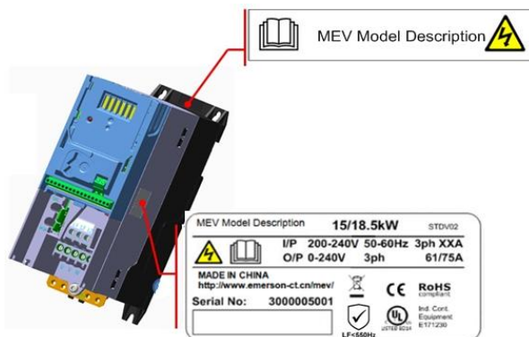
图A-1 图铭牌和条码位置示意图
