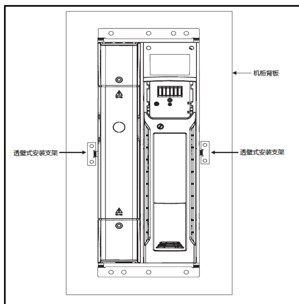
图 3-19 透壁式安装示意图
