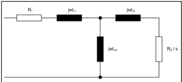
图 5-61 异步电机稳态等效电路图
