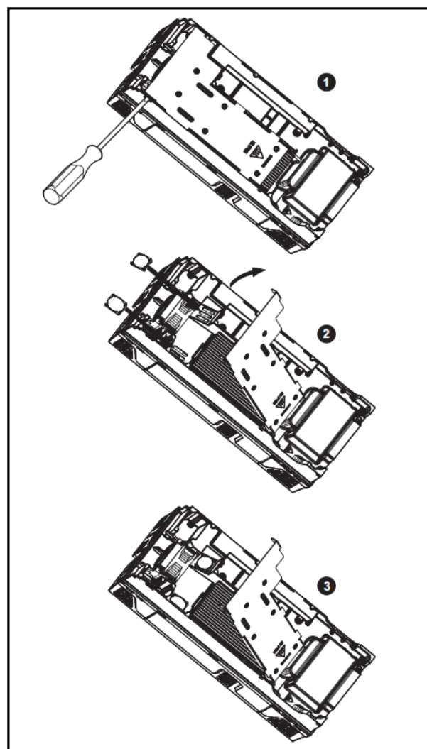
图 3-20 安装 IP 插片
