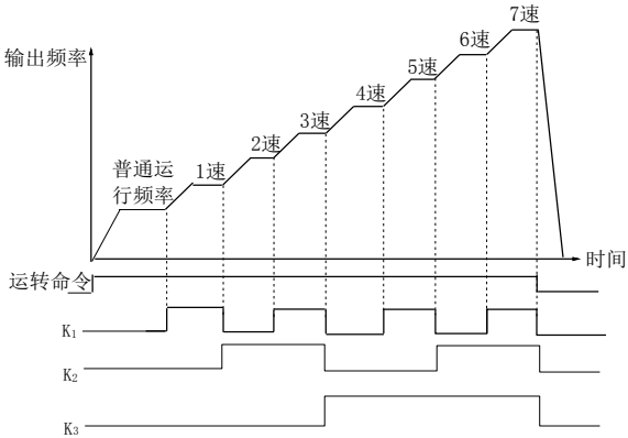
图 5-34 多段速度运行示意
