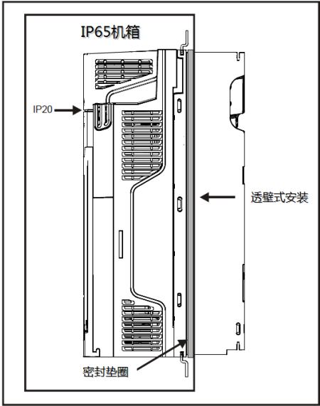
图 3-17 IP65 等级的柜内安装图
