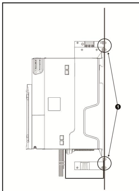
图 3-50 变频器，电机线缆屏蔽和滤波器接地
