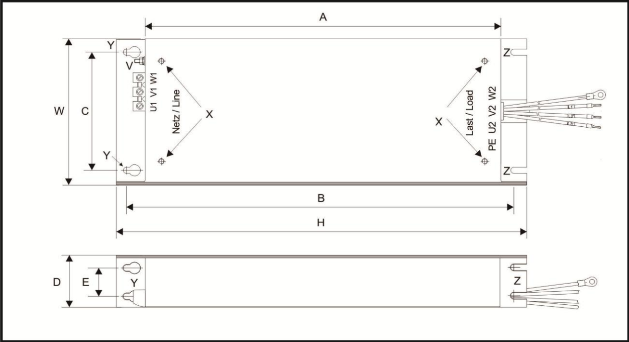
附图 4 EMC 滤波器外形尺寸 Size1 to 6
