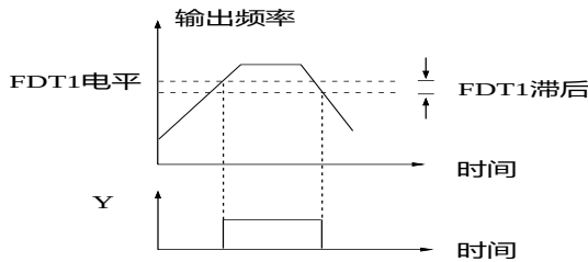
图 5-43 频率水平检测示意图
