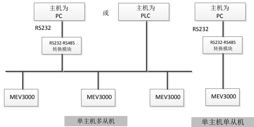
附图 7 变频器组网方式示意图
