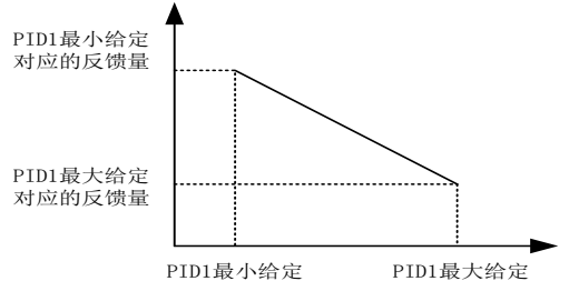
图 5-27 给定、反馈曲线示意图
