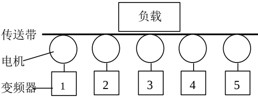
图 5-49 下垂控制示意图
