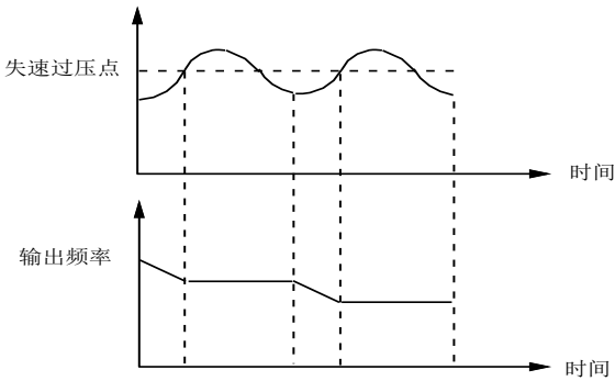
图 5-62 过压失速功能
