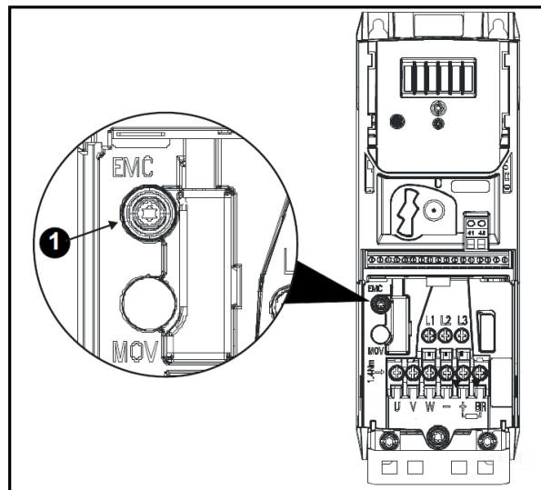
图 3-39 Size2-4 内置 EMC 滤波器移除示意图
