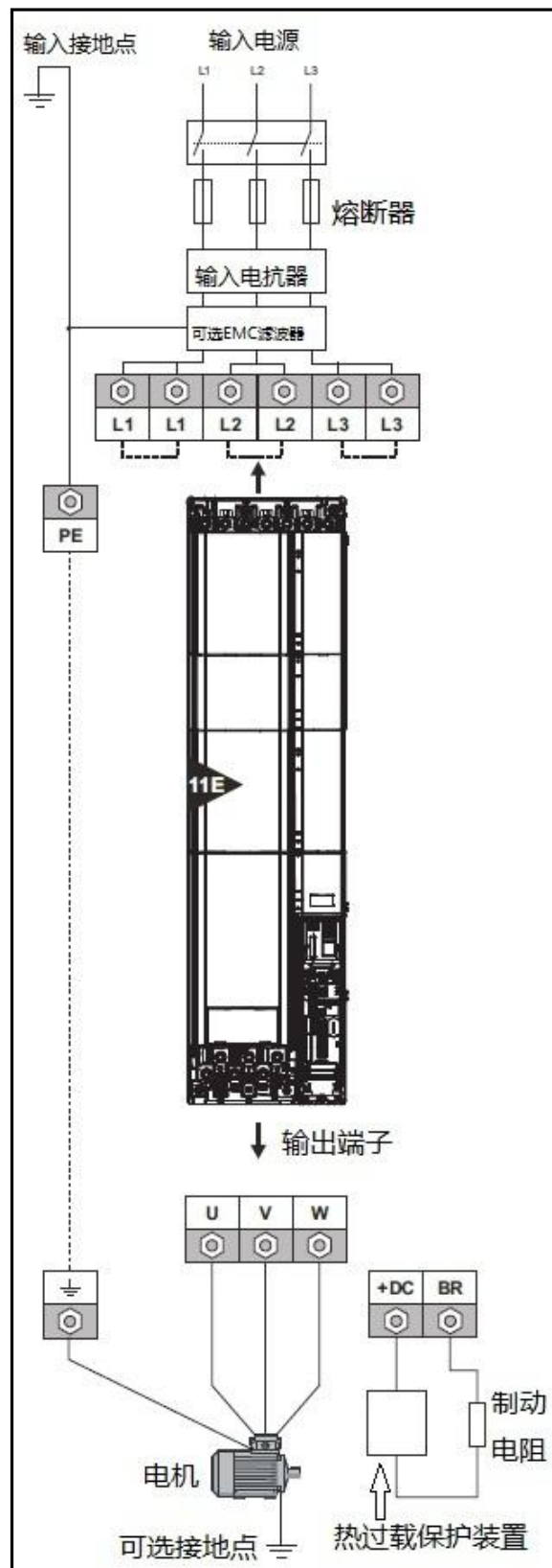
图 3-31 Size11 主回路输入输出连接图
