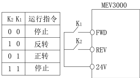
图 5-38 两线式运转模式 1
