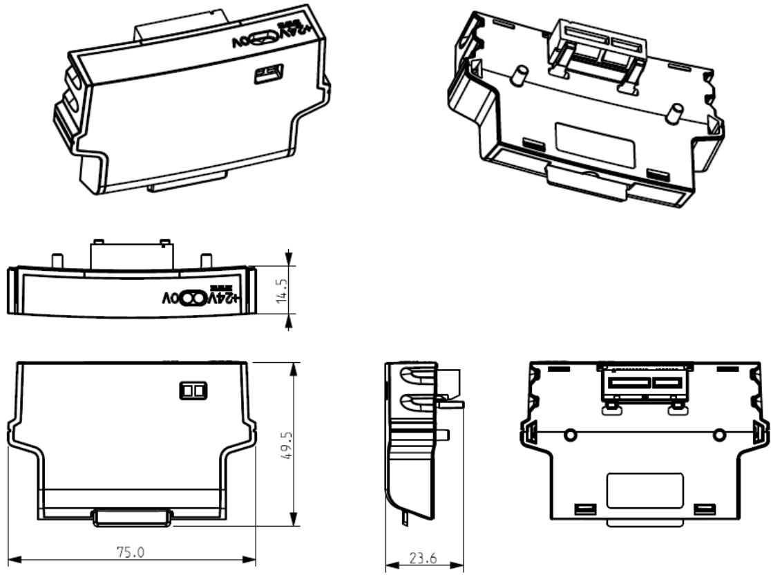
图 2-8 SD 卡适配器尺寸
