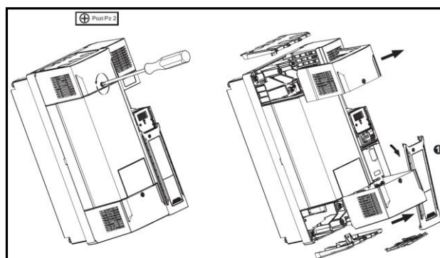
图 3-3 Size5 ~ 11 盖板拆卸示意图
