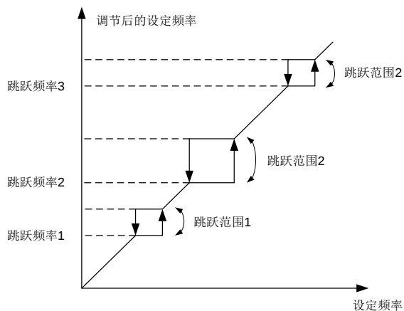
图 5-16 跳跃频率及范围示意图
