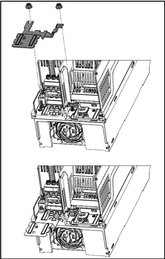
图 3-37 Size5 接地夹钳安装示意图
