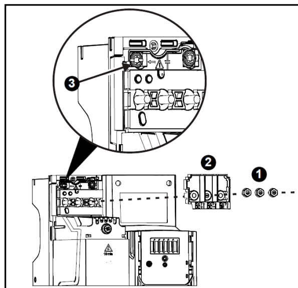
图 3-40 Size5 内置 EMC 滤波器移除示意图
