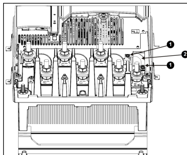
图 3-44 Size11 内置 EMC 滤波器移除示意图
