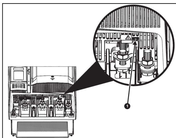
图 3-43 Size10 内置 EMC 滤波器移除示意图
