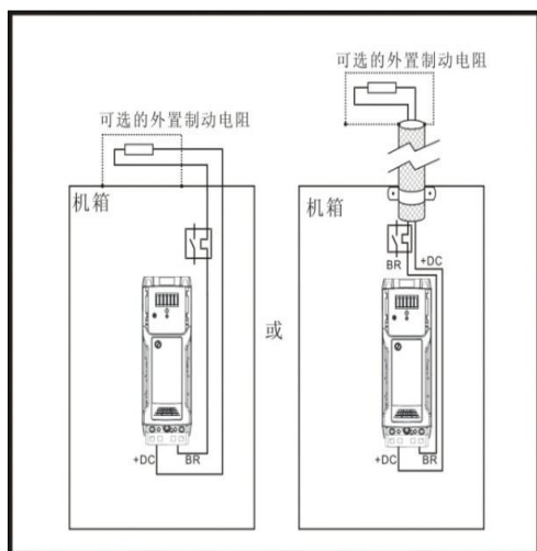
图 3-52 可选外置制动电阻器的屏蔽要求
