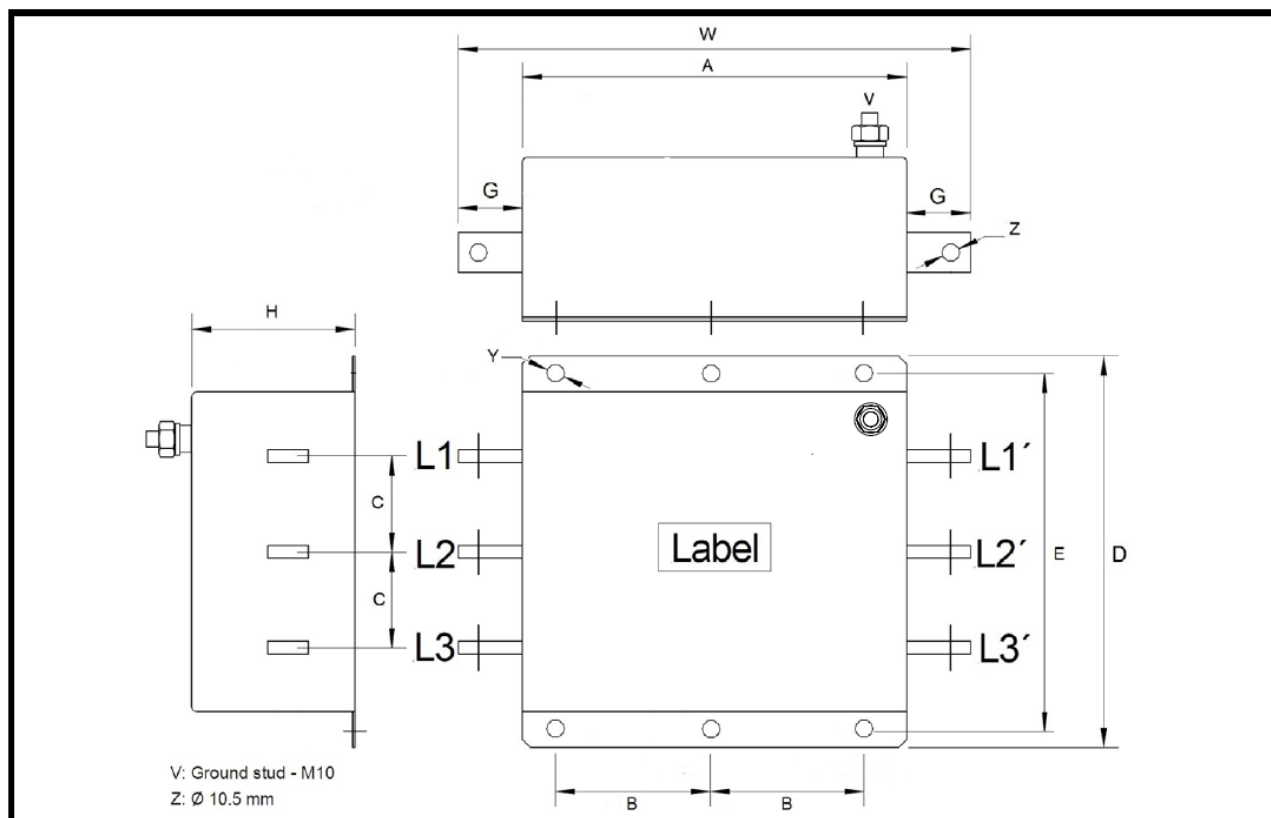
附图 6 EMC 滤波器外形尺寸 Size 9~11
