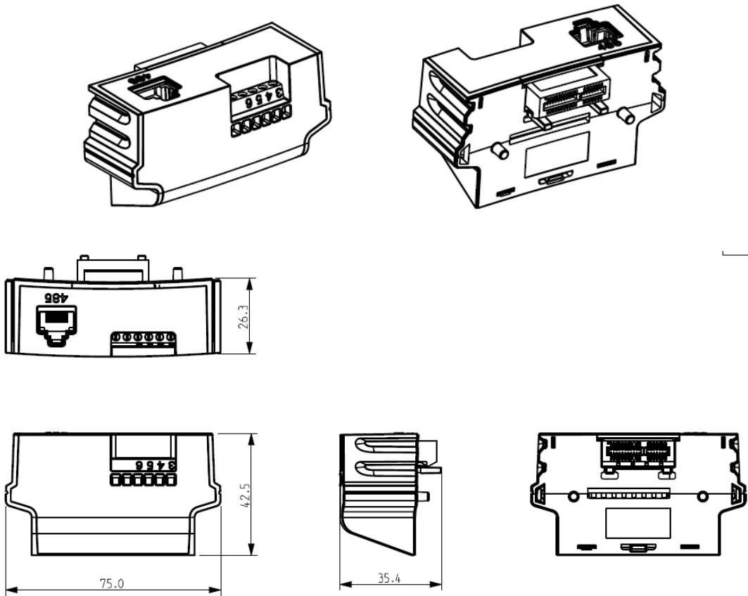
图 2-7 外置 RS485 适配器尺寸
