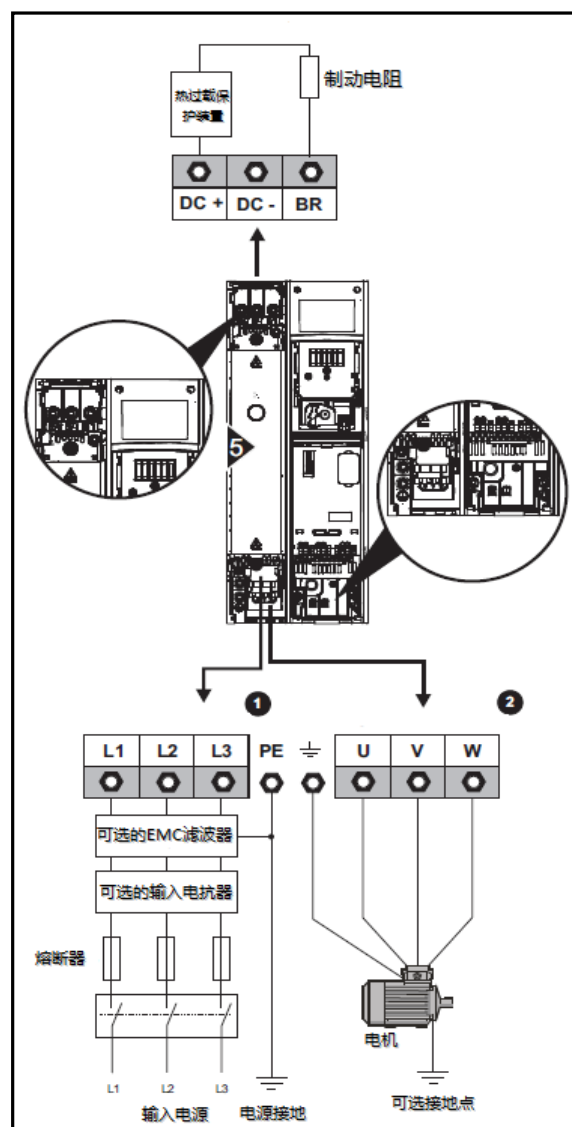
图 3-27 Size5 主回路输入输出连接图
