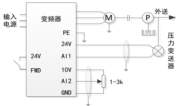
图 5-22 内置 PI 模拟反馈控制系统示意图
