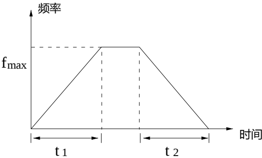
图 5-11 直线加减速
