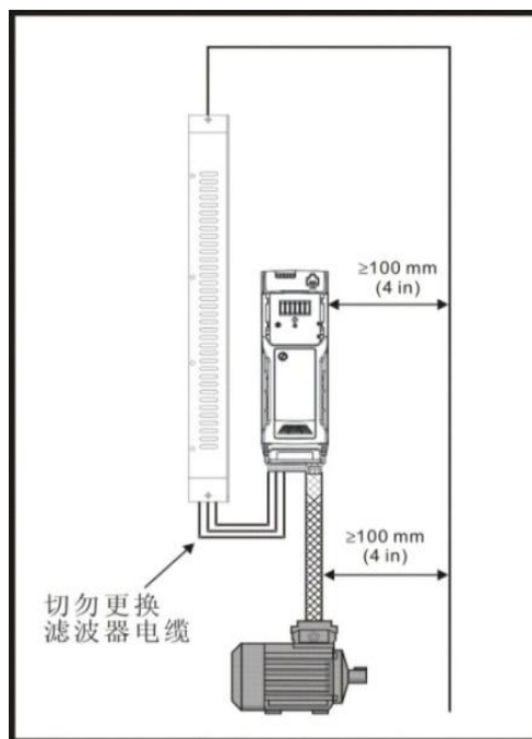
图 3-47 电源及接地线缆间距（Size2-6）
