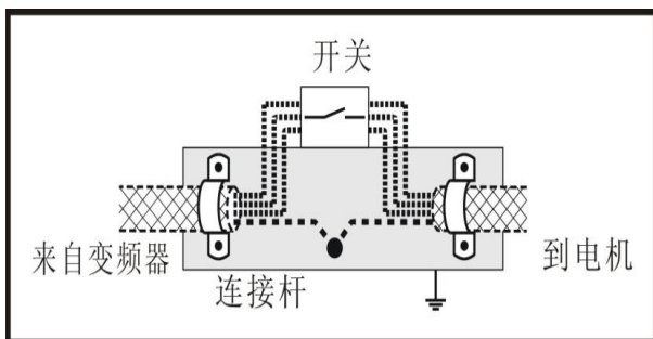
图 3-55 连接电机电缆至隔离开关
