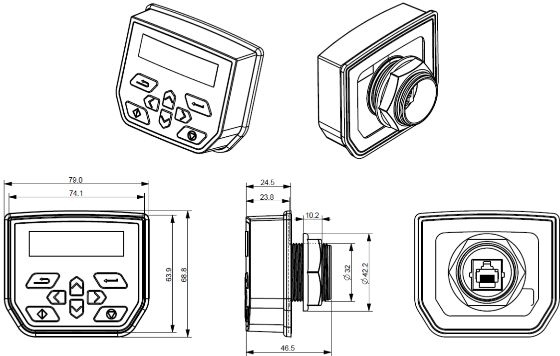
图 2-6 远程键盘尺寸
