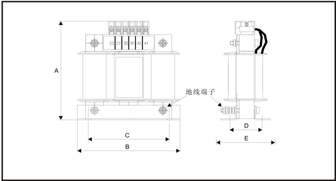
附图 2 交流输入电抗器外形图（4402-0227，4402-0228，4402-0229）
