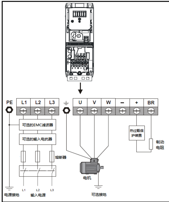
图 3-24 Size2 主回路输入输出连接图
