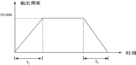
图 5-1 加减速时间定义
