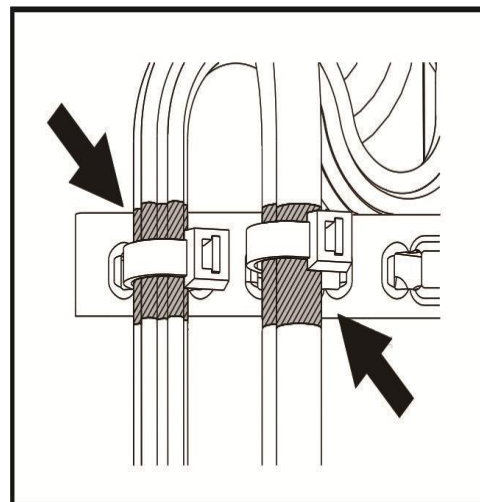
图 3-53 使用接地支架进行信号线缆屏蔽接地
