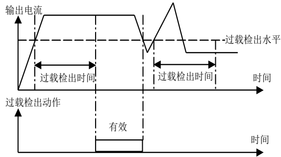
图 5-63 过载预警检出功能示意图
