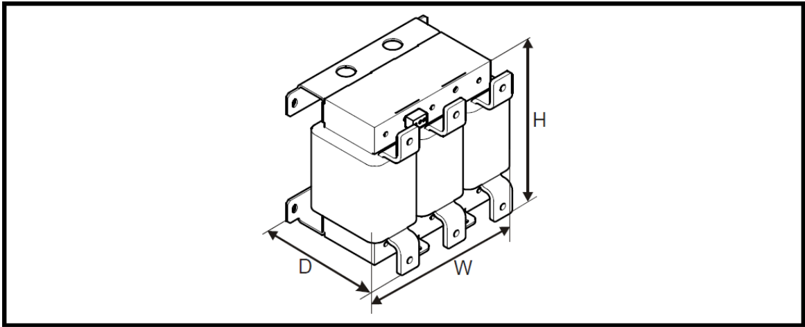
附图 3 交流输入电抗器外形图（4401-0227，4401-0228，4401-0229）
