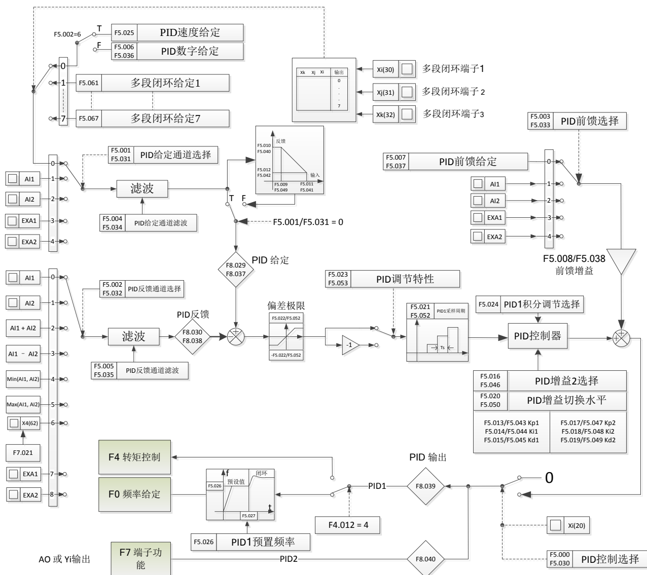
图 5-24 PI 原理示意图
