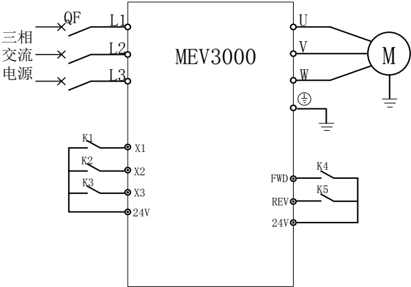
图 5-35 多段速度运行连接图
