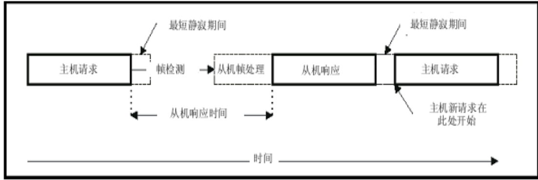
附图 9 主从通讯时间示意图
