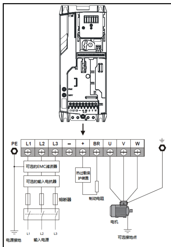
图 3-26 Size4 主回路输入输出连接图
