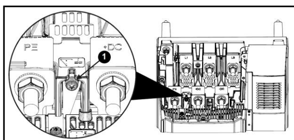
图 3-42 Size7-9 内置 EMC 滤波器移除示意图
