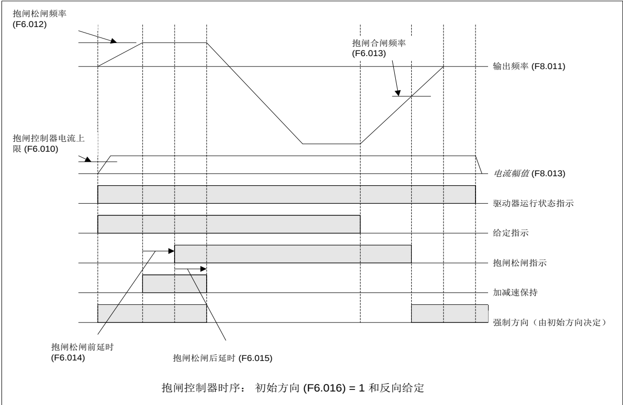
图5-33 抱闸控制器时序：初始方向（F6.016）=1和反向给定
