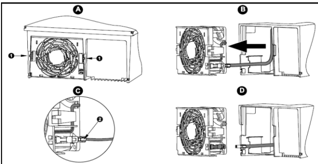
图 3-22 风扇拆除示意图
