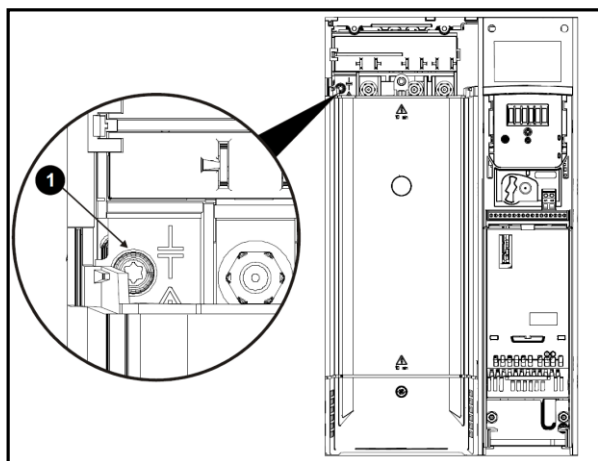
图 3-41 Size6 内置 EMC 滤波器移除示意图
