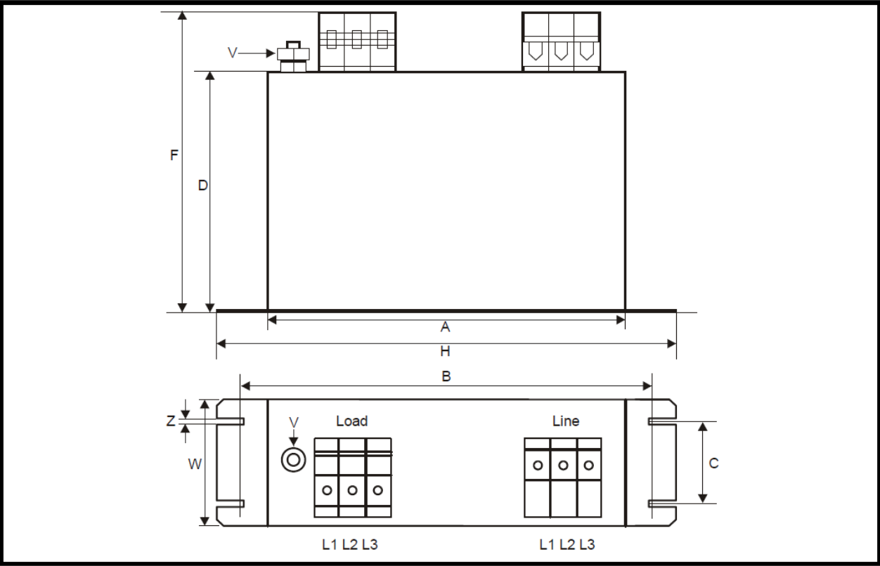
附图 5 EMC 滤波器外形尺寸 Size7~8
