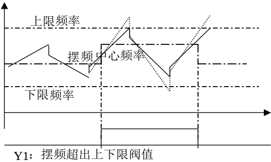
图 5-37 摆频幅度限制
