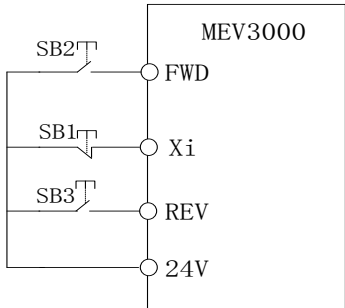
图 5-40 三线式运转模式 1
