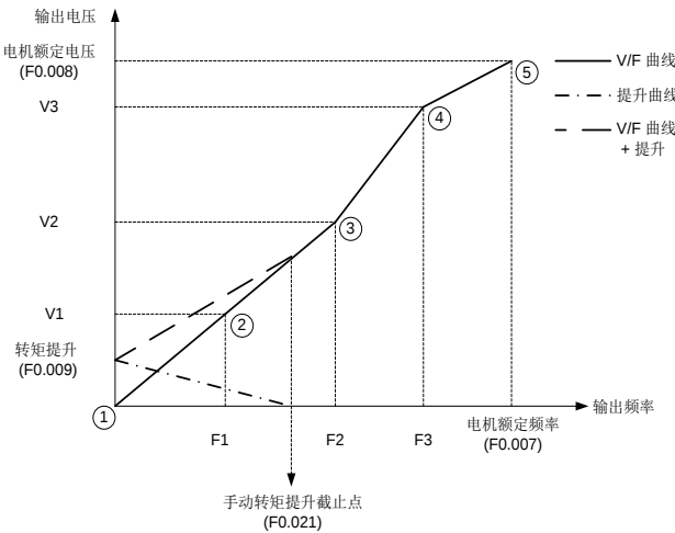
图5-3 自定义V/F曲线
