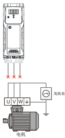
图 1-1 电机绝缘检查示意图
