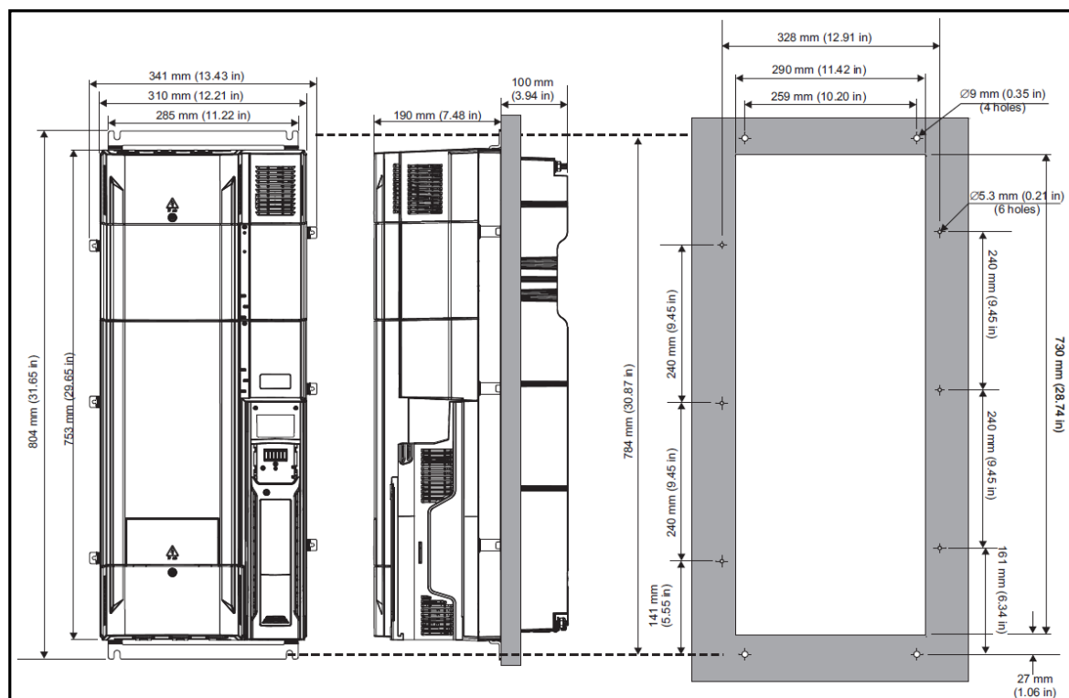
图 3-14 Size8 透壁式安装尺寸图
