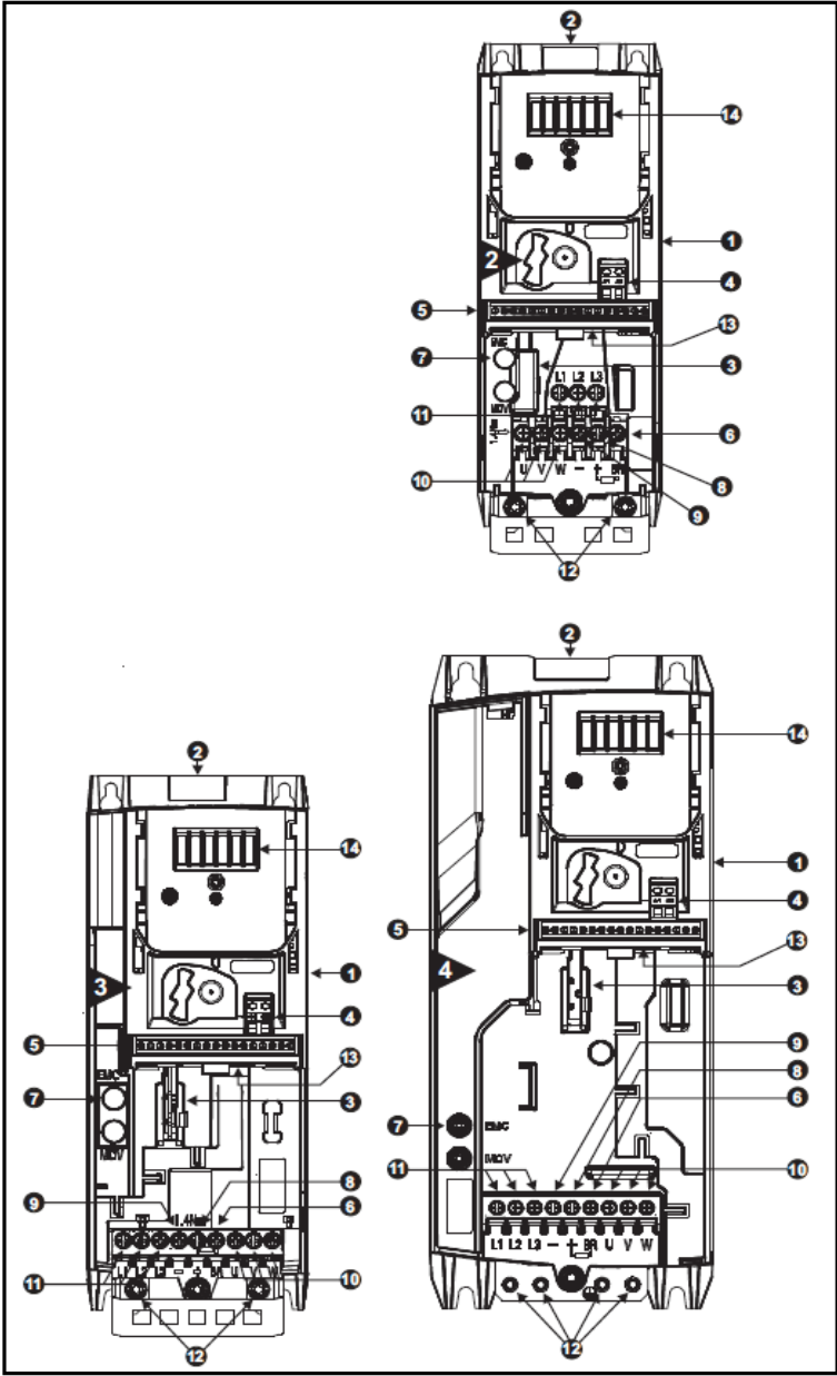
图 2-1 Size 2~4 (0.37kW - 7.5kW)变频器各部位名称示意图
