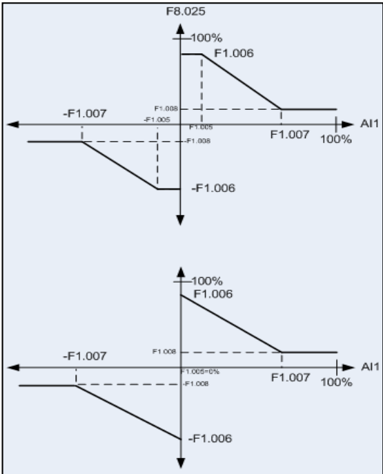
图 5-7 模拟输入 AI1 给定反作用特性
