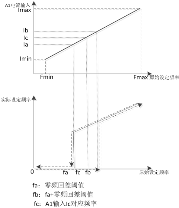
图 5-51 零频回差运行
