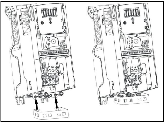
图 3-35 Size2-4 接地支架安装示意图
