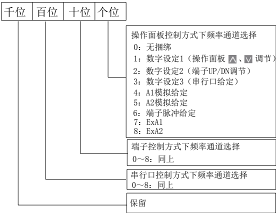
图 5-46 运行命令通道捆绑频率给定通道
