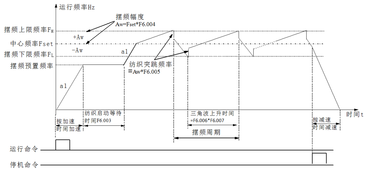
图 5-30 摆频示意图
