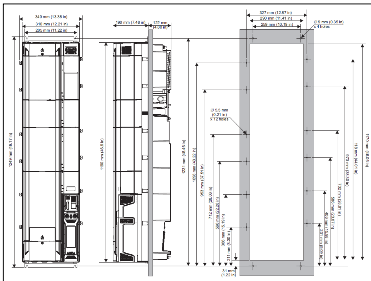
图 3-16 Size11 透壁式安装尺寸图
