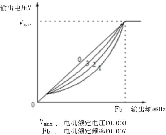
图5-2 降转矩曲线
