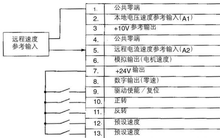
图 6.5 端子连接
