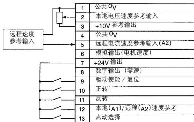
图 6.3 端子连接
