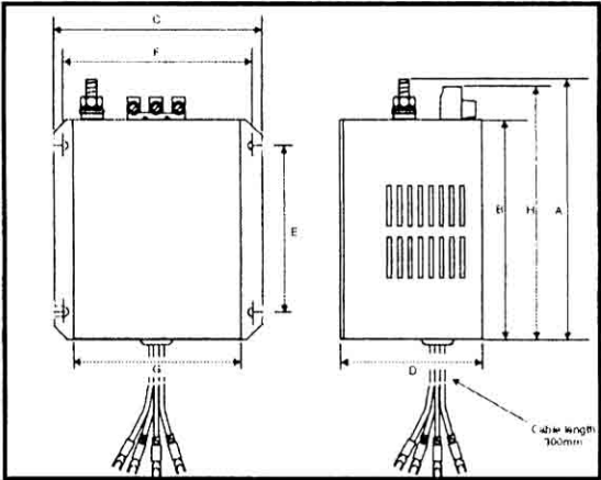
图 4.10 RF1滤波器尺寸
