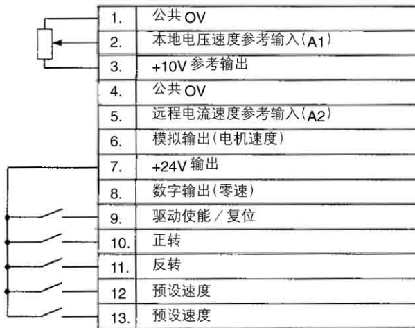
图 6.4 端子连接
