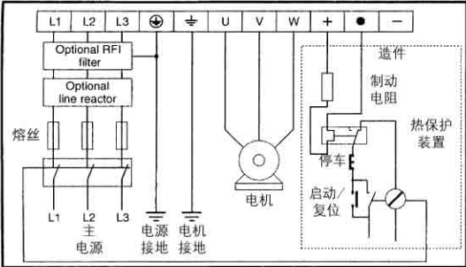
图5.3 Commander SE规格5电源端子接线图
