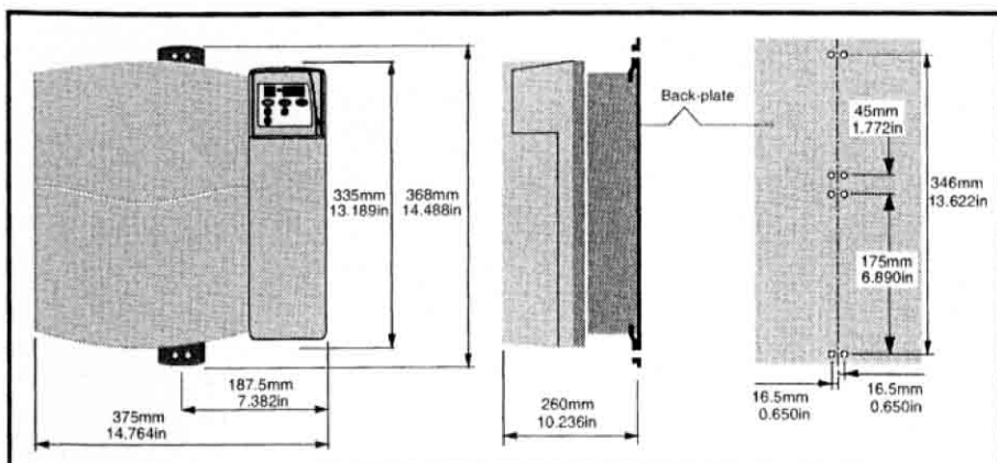
图 4.4 规格 5 单元表面安装图
