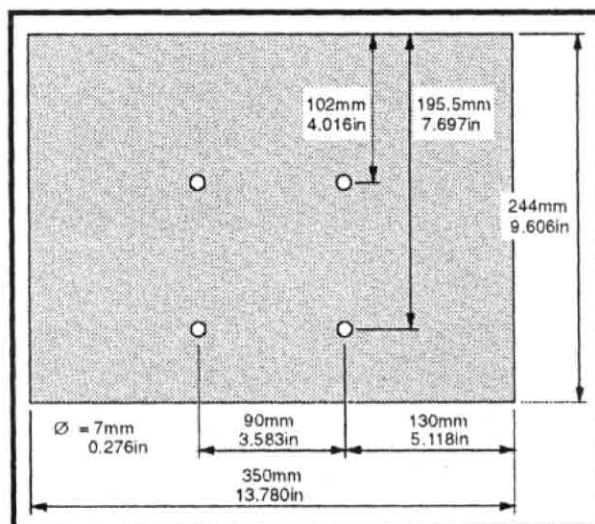
图 4.7 规格 5 挡板
