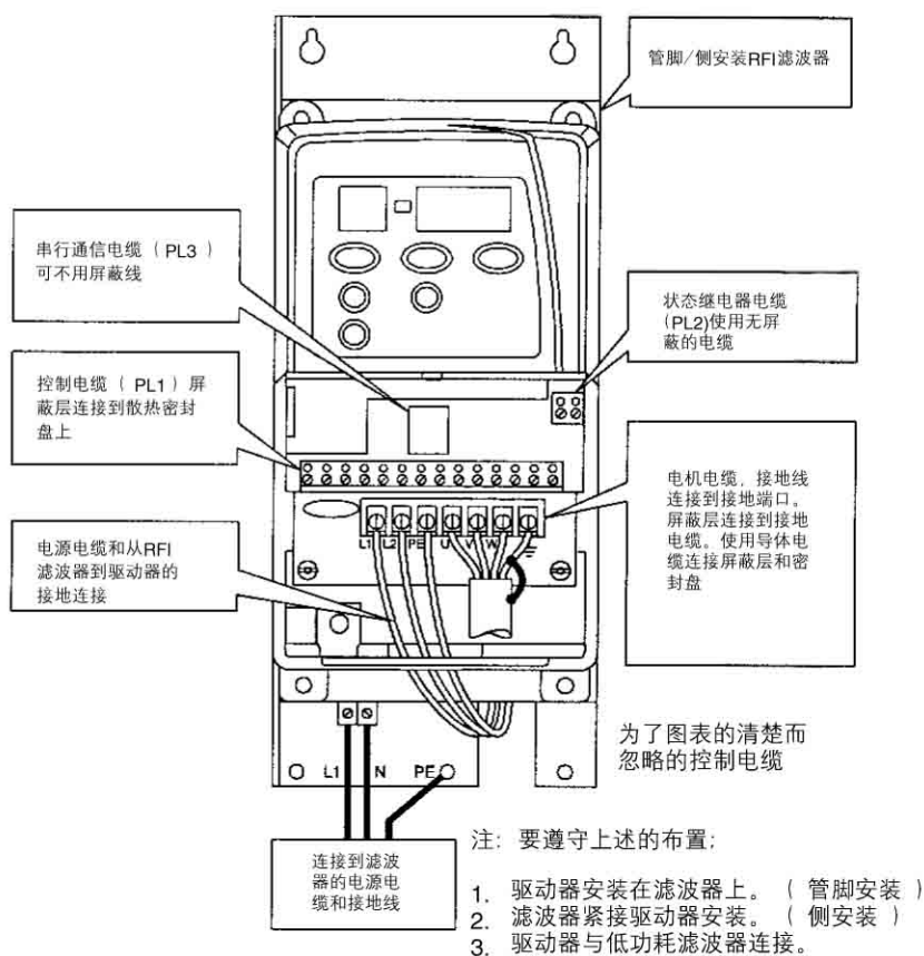
图4.14 完善的EMC措施
