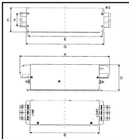
图 4.11 RF1滤波器尺寸
