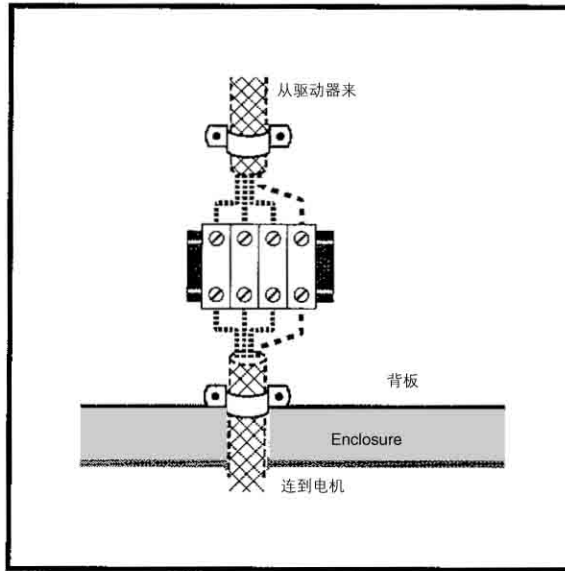
图 4.15 连接电机电缆和密封壳内的端子区
