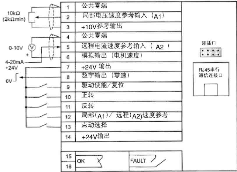
图 5.4 控制端口连接
