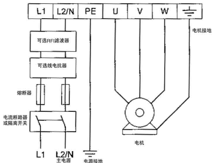
图5.1 Commander SE规格1电源端子接地
