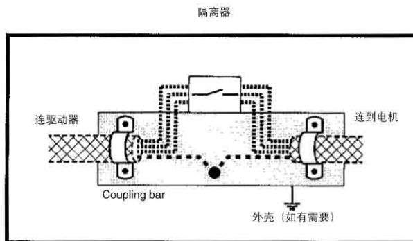
图 4.16 连接电机电缆和隔离开关
