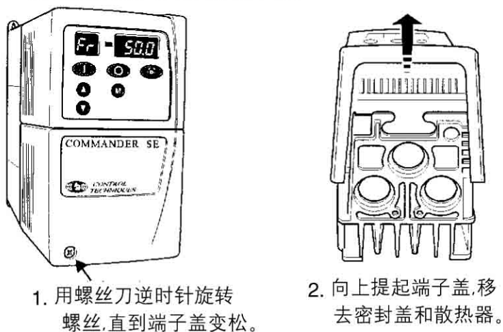
图 4.1 规格1 打开驱动器端子盖
