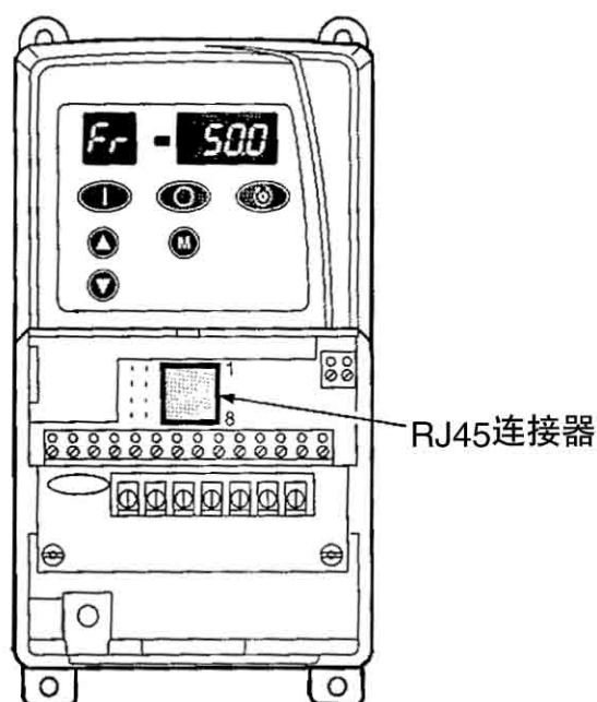
图9.1 连接图
