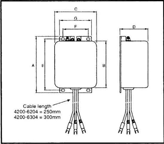
图 4.9 RF1滤波器尺寸
