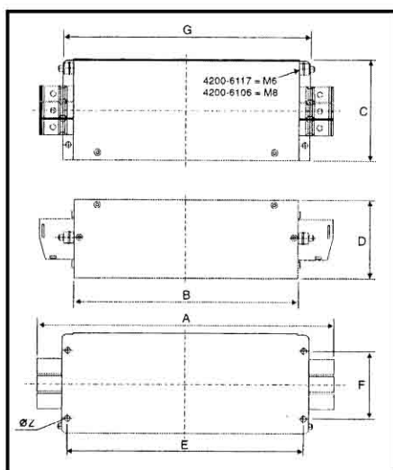
图 4.12 RF1滤波器尺寸
