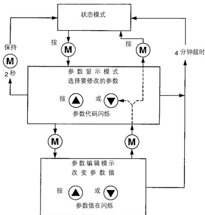
图 6.2 (第 53 页)选择和修改参数
