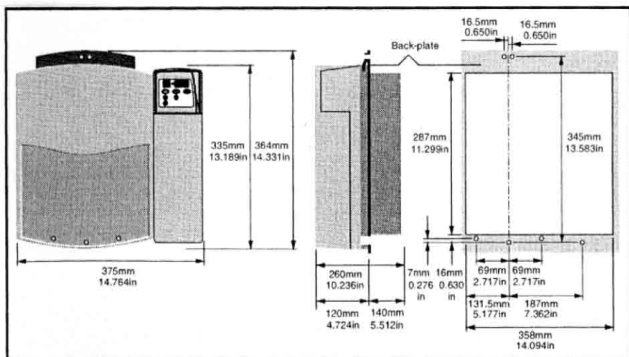
图 4.5 规格 5 单元开孔安装图
