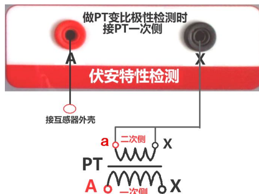
图 23, PT 交流耐压接线图
