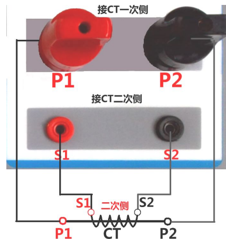
图 11 , CT 变比极性接线图
