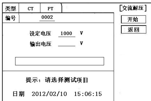
图 15, CT 交流耐压测试界面
