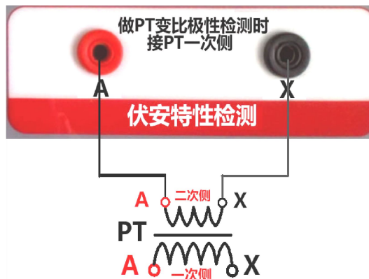
图 18, PT 励磁特性接线图
