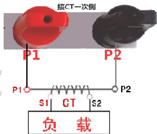
图 14、CT 一次通流接线图
