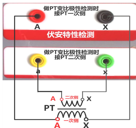
图 20 , PT 变比极性接线图
