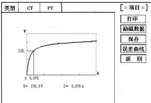
6, CT 励磁曲线图
