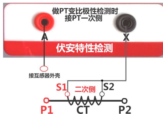
图 16, CT 交流耐压接线图
