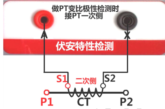
图 5, CT 励磁特性接线图
