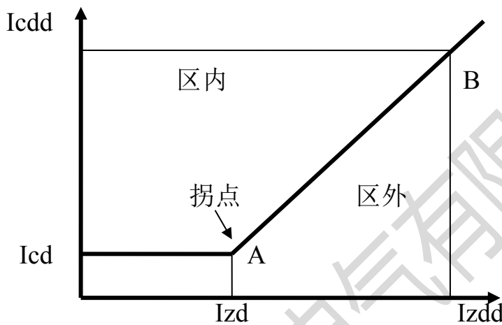
图 1 为微机型差动保护的比率制动特性曲线
