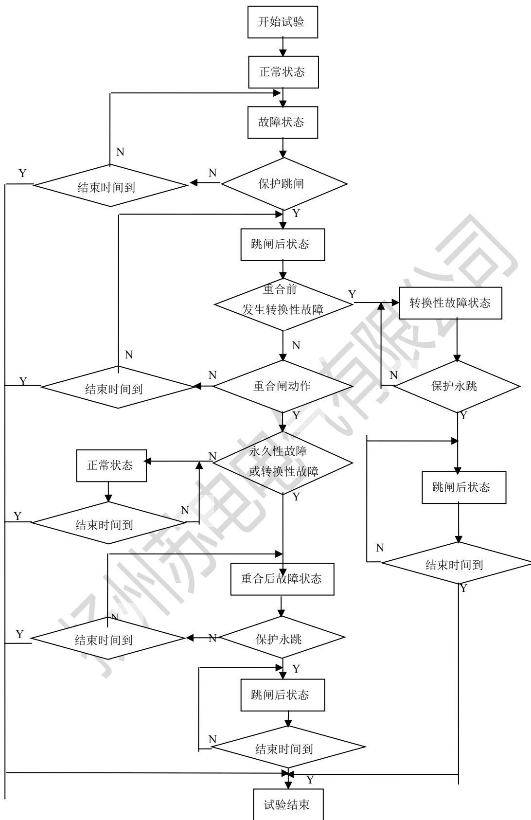
整组传动试验程序框图如下所示：
