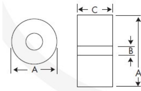
红宝石气阻尺寸图
