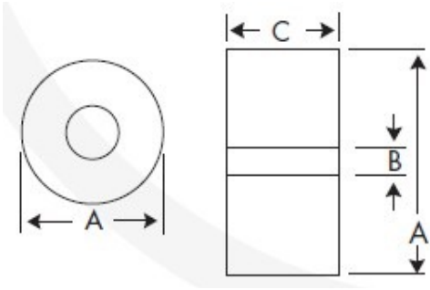
0.118外径红宝石外型尺寸图
