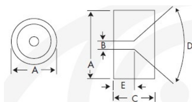
蓝宝石气阻尺寸图
