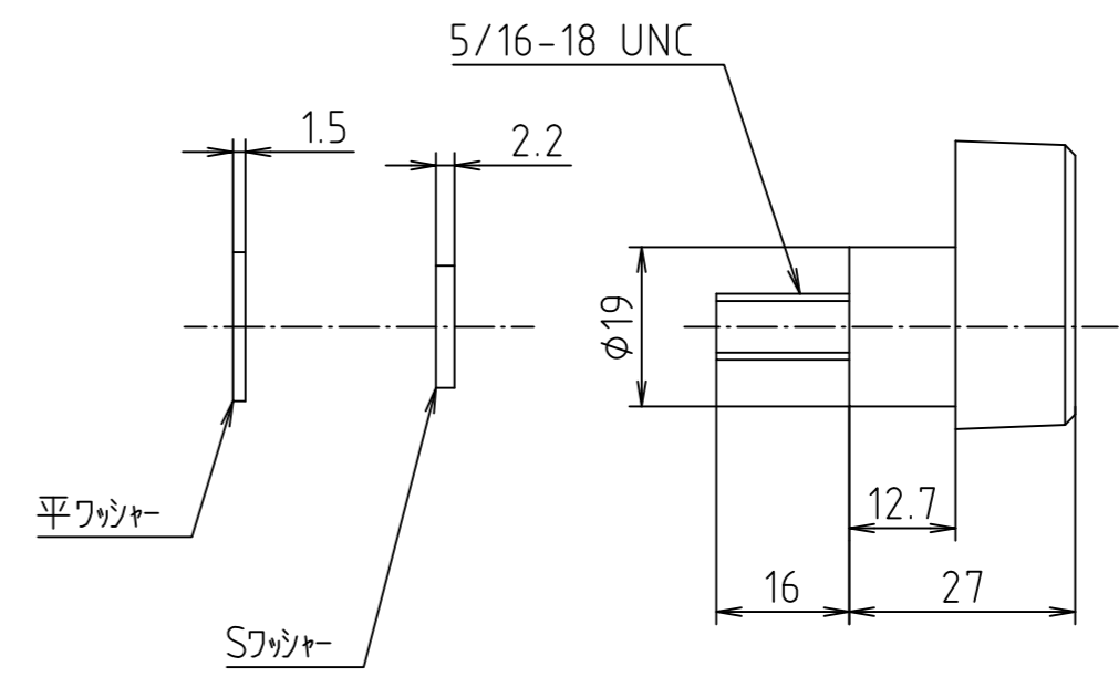
ノズル詳細 (S=1/1)
