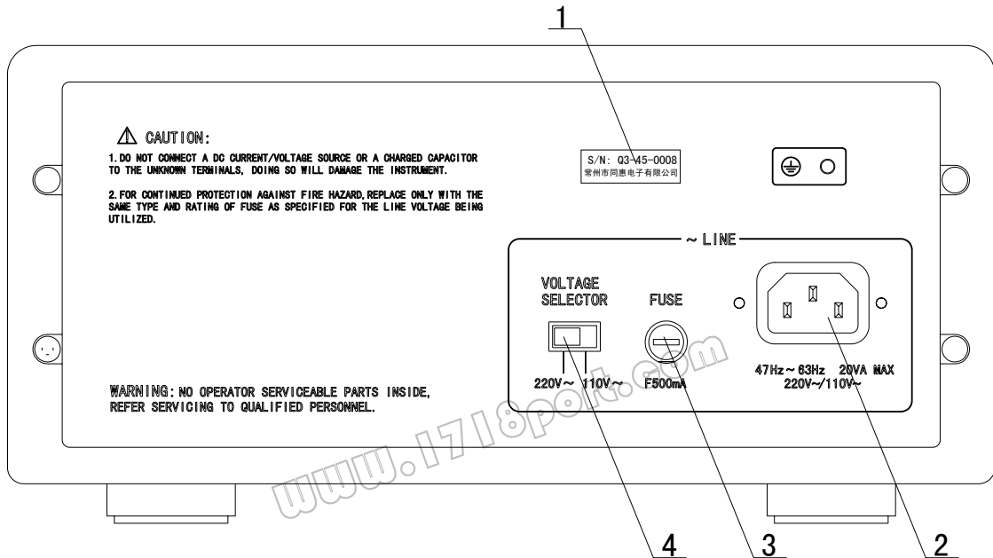
图 2-2. 后面板
