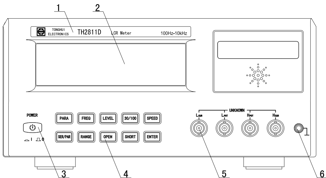
图 2-1. 前面板
