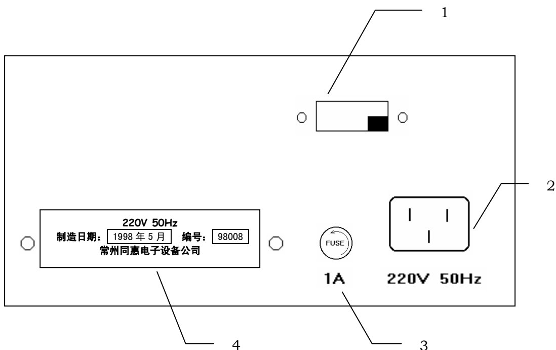
图 1-2 后面板图
