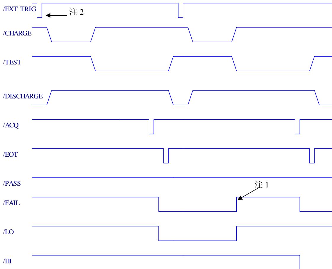
图 7-2 SEQ.TEST 时序
