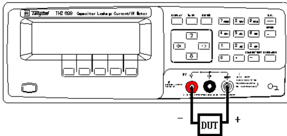
图3-1 被测件连接图
