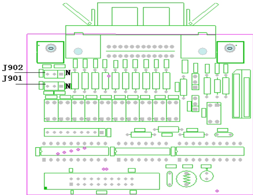
图 7-1 跳线
