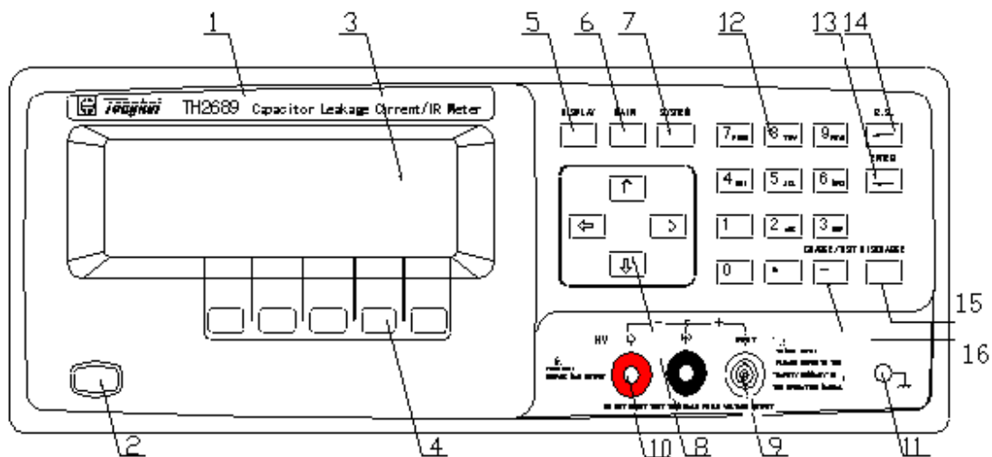
图2-1 仪器前面板示意图
