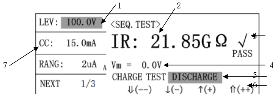
图 3-3 (a) SEQ.TEST 第一页选项
