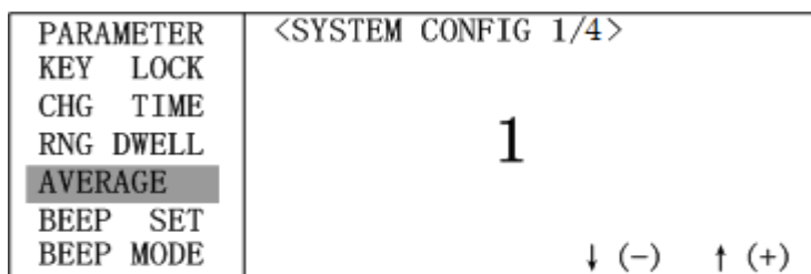
图 3-35 测量平均次数的设置
