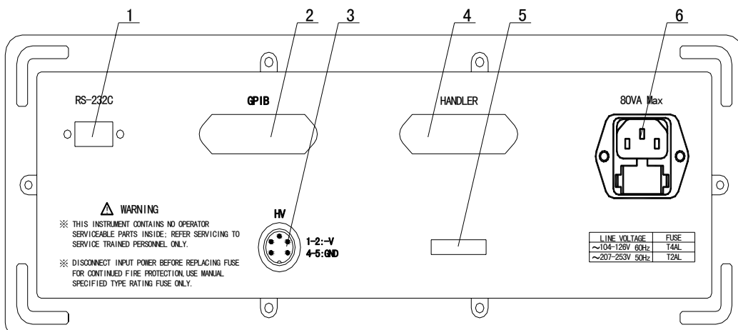
图 2-2 仪器后面板示意图
