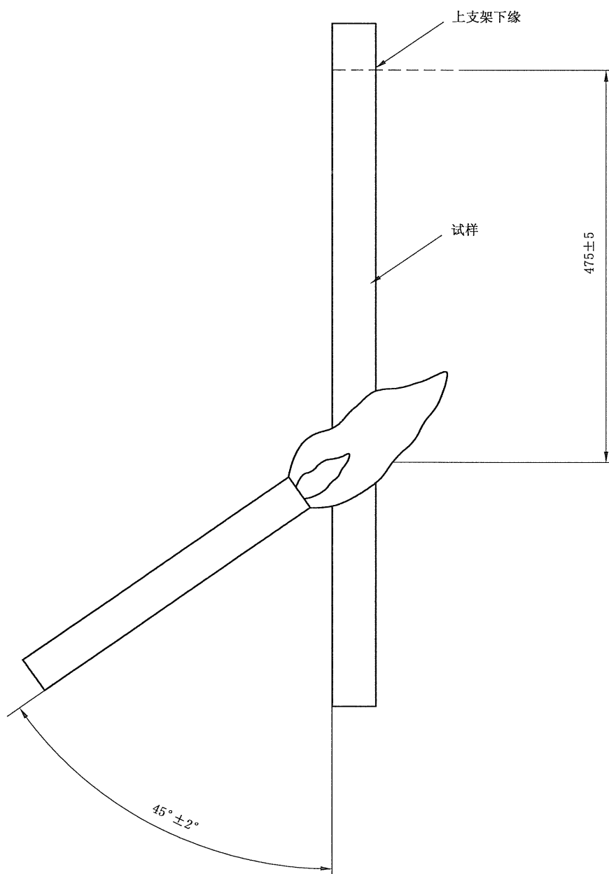
图 2 对试样供火
