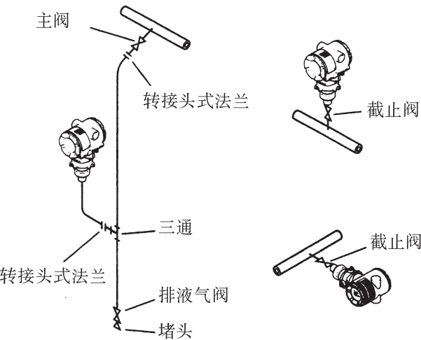
图 5.2 引压管连接示例
