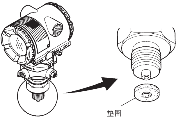
图 4.2.2 垫圈
