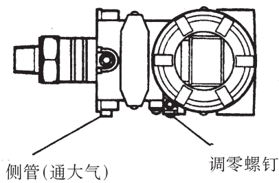
图 5.1.1 水平配管连接
