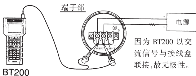
图 6.3.3 BT200 的连接
