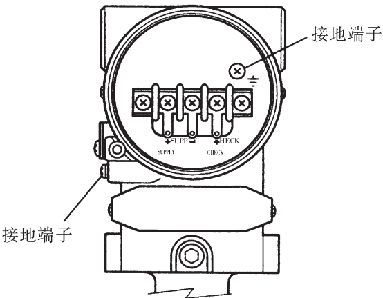
图 6.5 接地端子
