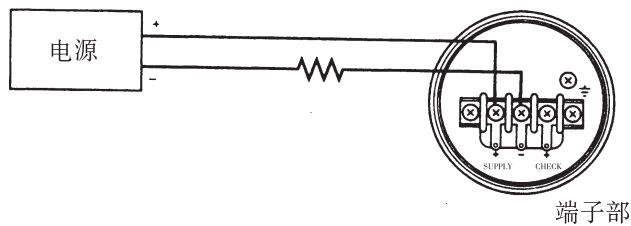
图 6.3.1 电源连接
