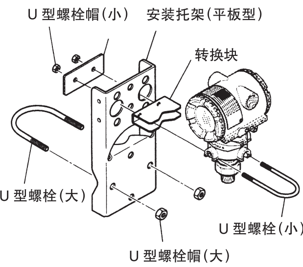
图 2.1.1 变送器安装部件
