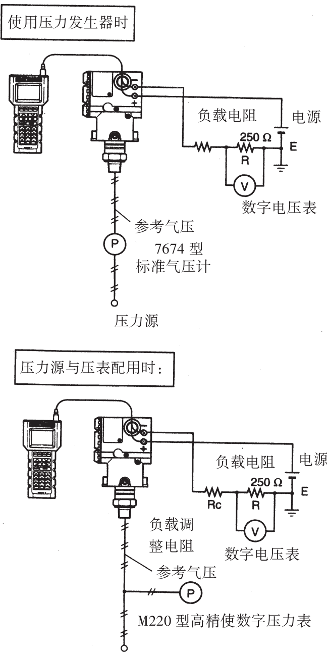
图 9.3.1 仪表连接
