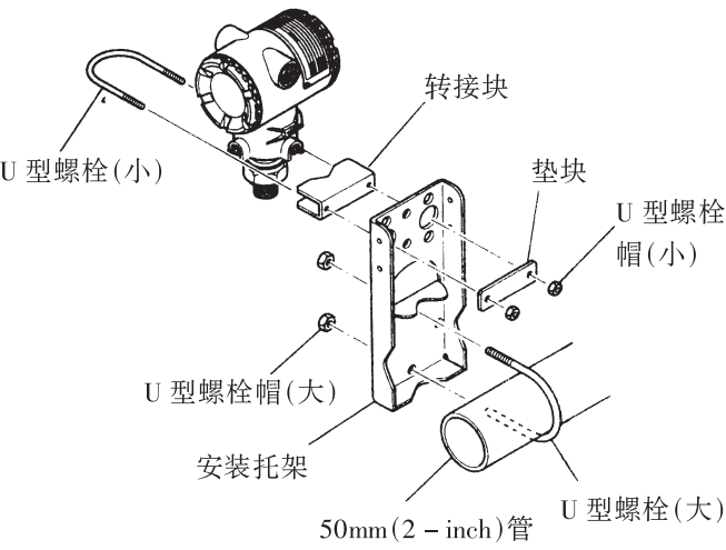
图 4.2.1 变送器安装
