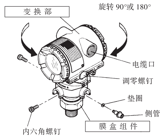
图 4.3 旋转变送部
