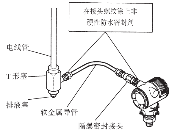
图 6.4.2b 用隔爆密封接头的典型配线
