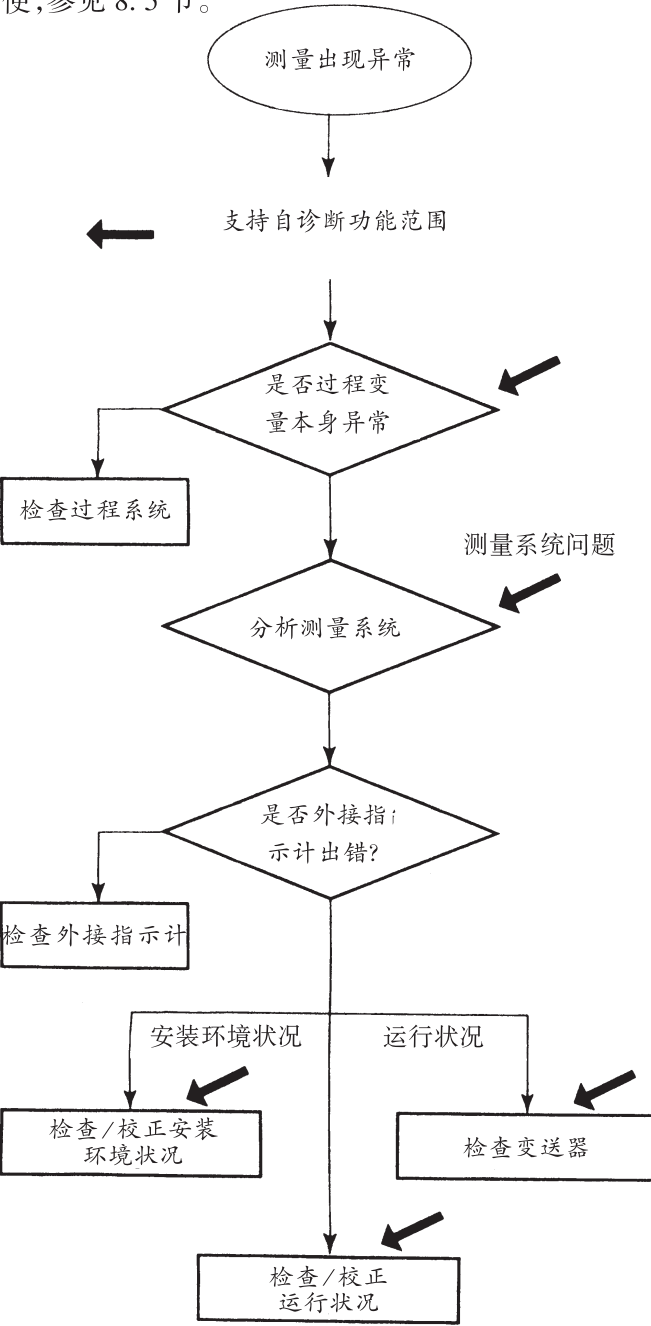
图 9.5.1 基本流程及自诊断
