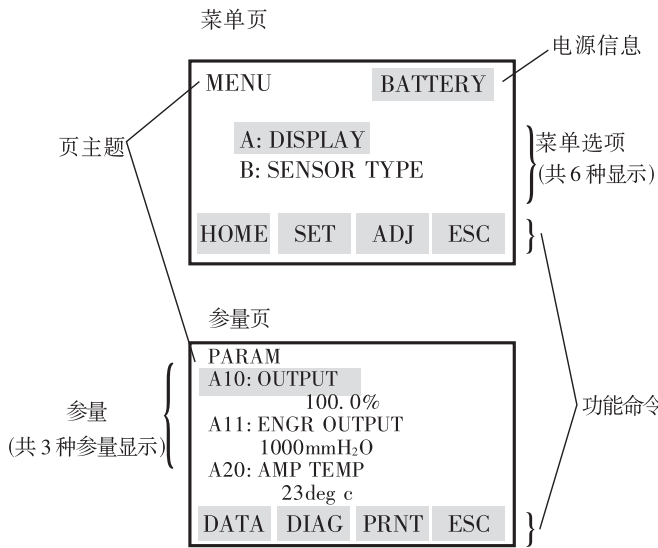
图 8.2.1 BT200 面图
