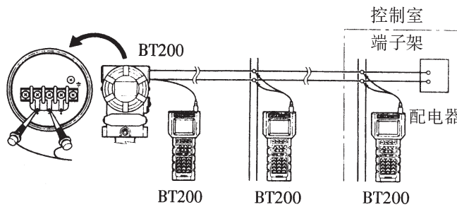
图 8.1.1 BT200 的连接
