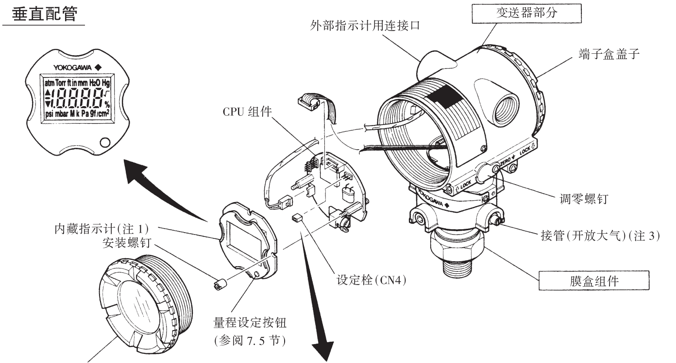
图 3.1 部件名称
