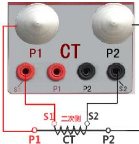
图 12, 电流法 CT 变比极性测试接线图
