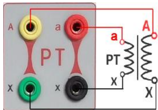
图 30, PT 变比极性（角差比差）接线图
