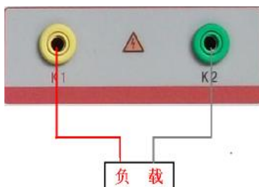
图 23, CT 二次负荷接线图
