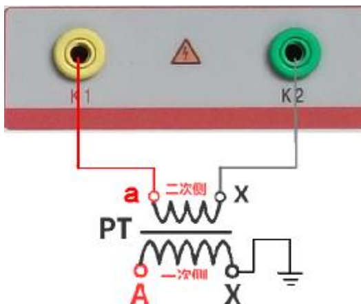
图 28，PT 励磁特性接线图
