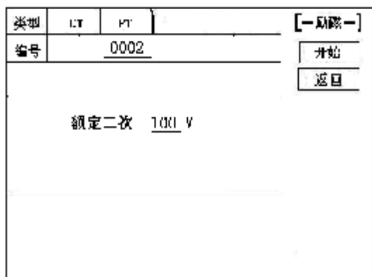
图 27，PT 励磁特性参数设置界面
