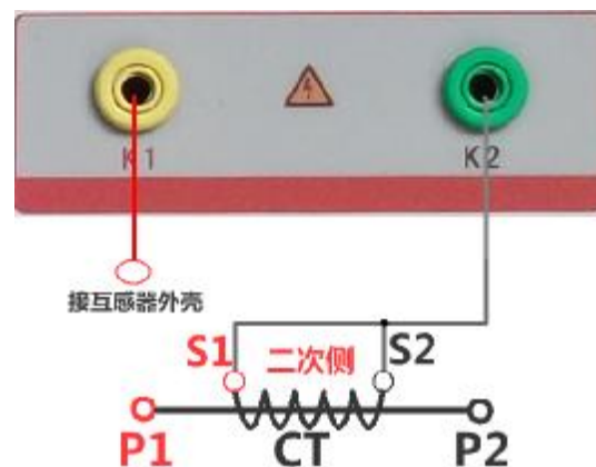
图 21，CT 交流耐压接线图
