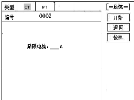
图 4, CT 励磁特性测试界面
