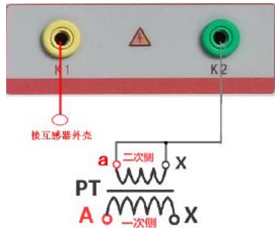
图 35，PT 交流耐压接线图
