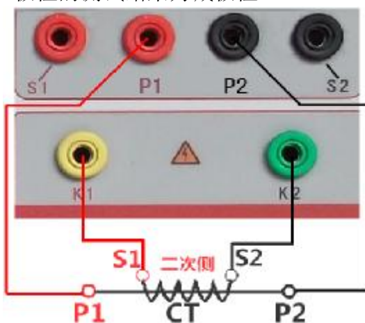
图 14, 电流法 CT 变比极性测试接线图
