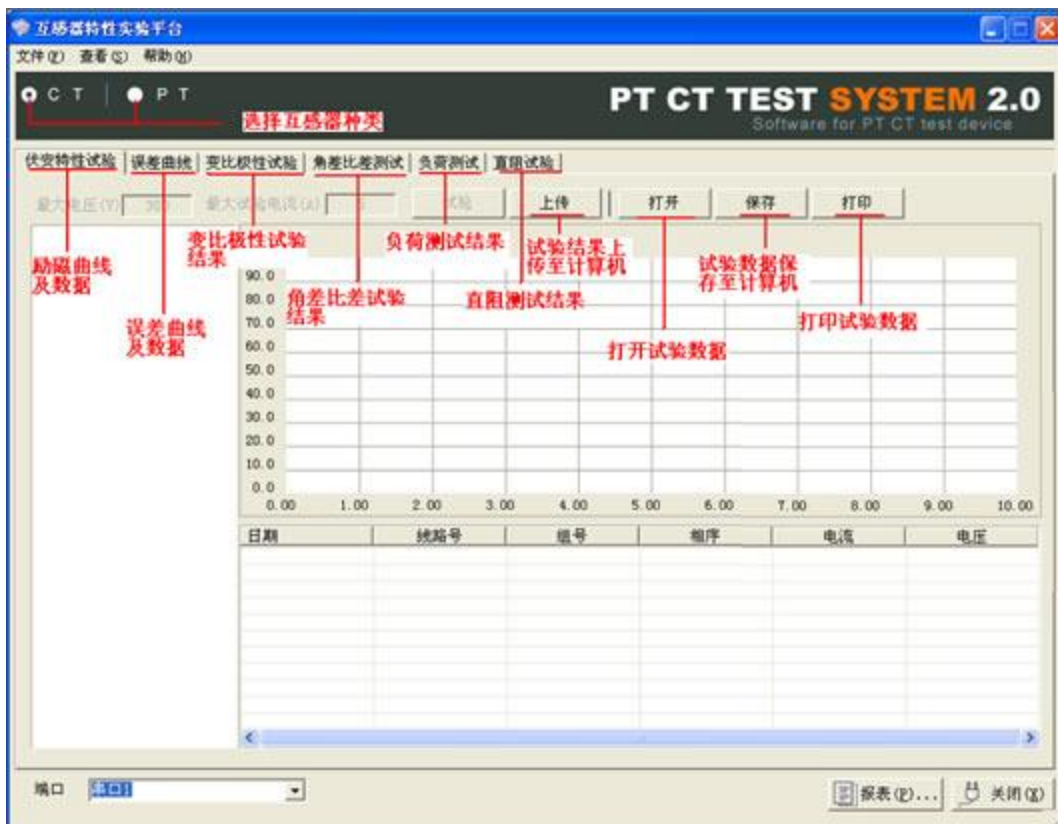
图 43，上位机操作软件
