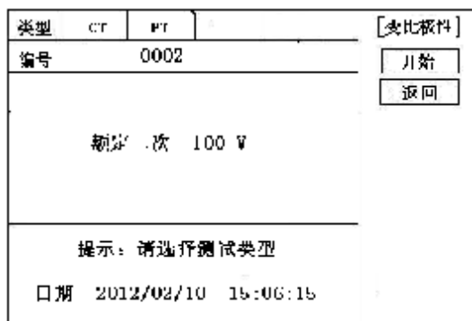
图 29, PT 变比极性测试界面
