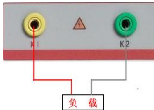
图 37，CT 二次负荷接线图
