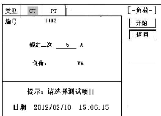
图 22, CT 二次负荷测试界面
