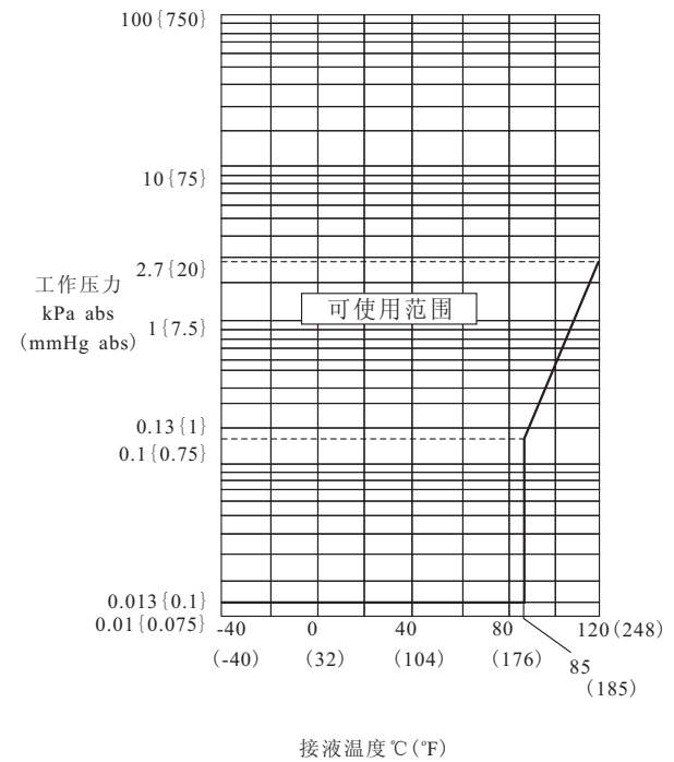
工作压力与环境温度关系图 [适用于 EJA530A]
