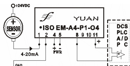
电流输入/电压输出 (I/V转换)
