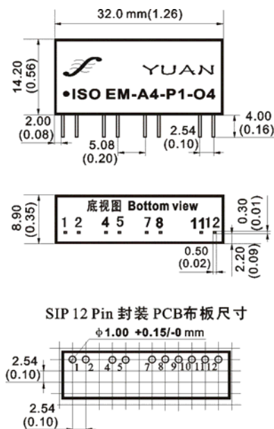
电流输入/电流输出 (I/I) 隔离
