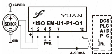
电压输入/电流输出 (V/I转换)
