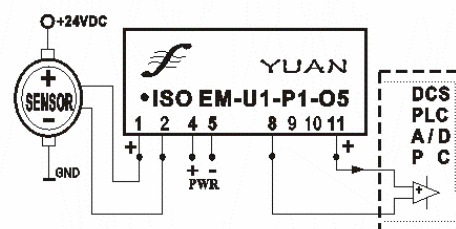
电压输入/电压输出 (V/V隔离)
