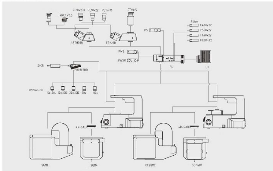
OMT-6R/OMT-6RT 系统配置图：
