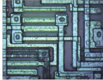
集成电路 100X 明场
