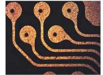
FPC 10X 暗场
