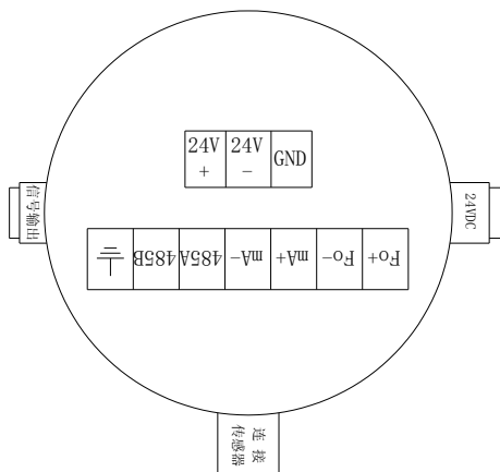
接线图
