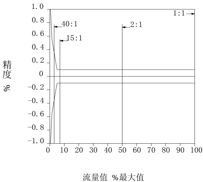
瞬时流量标准精度曲线
