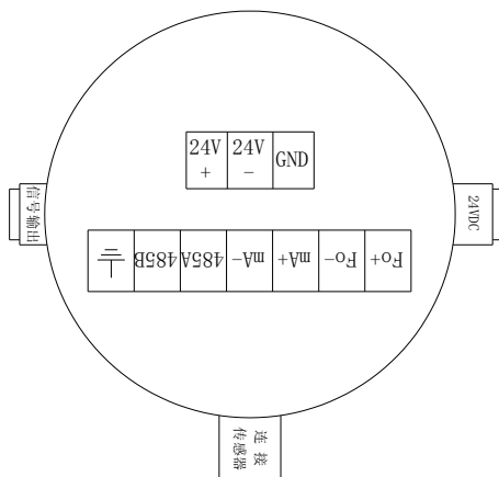
接线图
