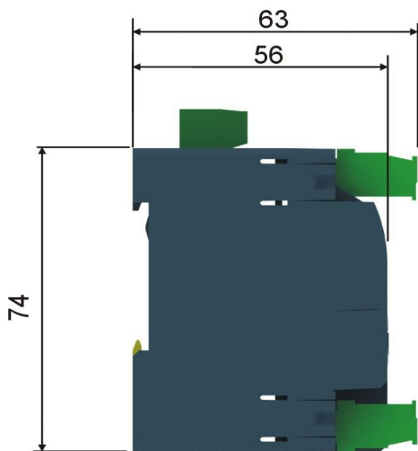
图 1 ZWD432B 安装尺寸图
