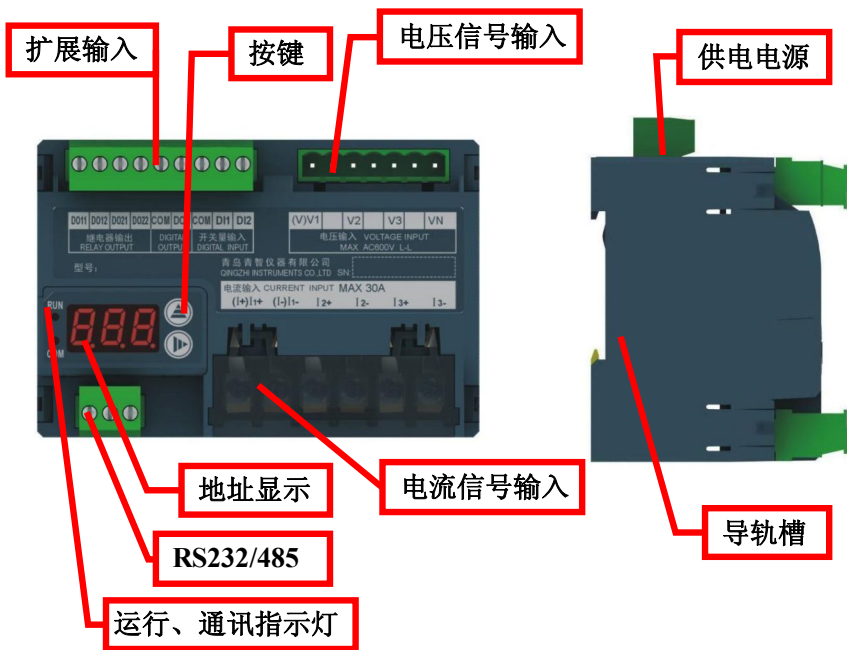
图 2 ZWD432B 实物图示
