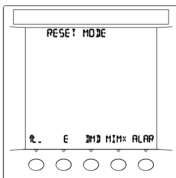
选择复位的参数
