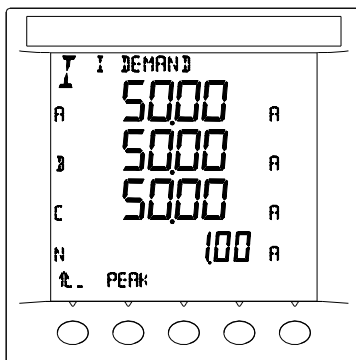
实时各相电流需量显示
