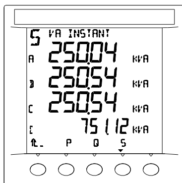
各相视在功率
