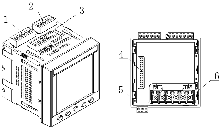
仪表连接端子
