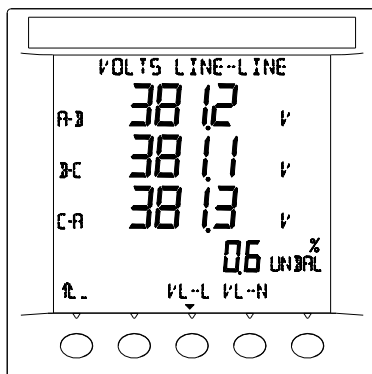
线电压及线电压不平衡度
