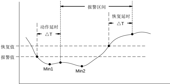
下限报警输出控制过程示意图
