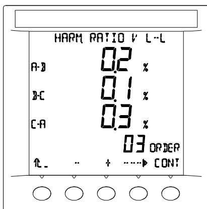
谐波含有率（当 ORDER \geq 01 时。如果 ORDER=01 显示的是基波含有率，为 100%）
