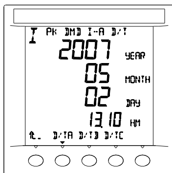
A 相电流需量峰值记录
