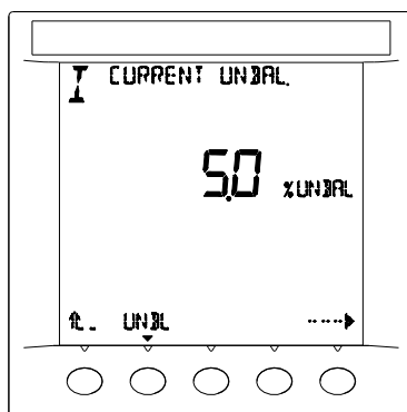
电流不平衡度
