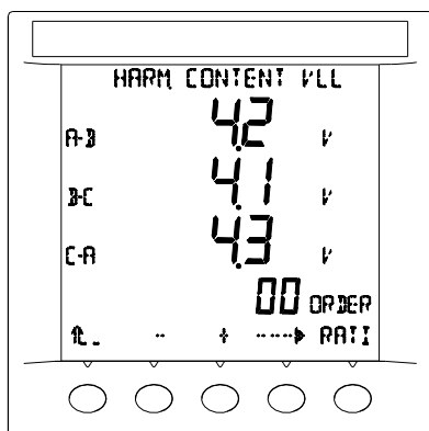
线电压谐波含量（当 ORDER=00 时）
