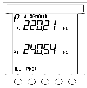
有功功率需量和峰值需量
