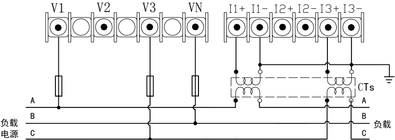
2-3. 三相三线系统，采用无 PT，2CT 方式的接线图（适用于 32 SYS，见 6.3.1 的设置仪表参数）
