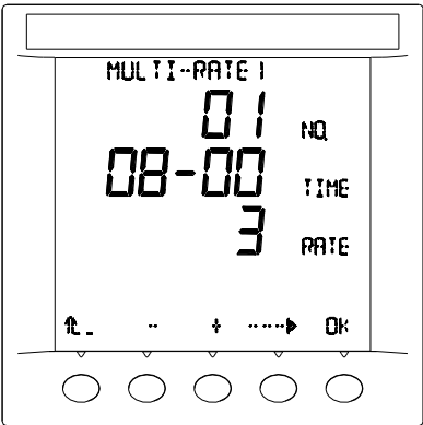
费率设置界面
