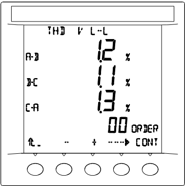
线电压总谐波畸变率（当 ORDER=00 时）
