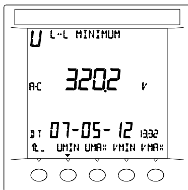
U: 线电压最小值及发生日期时间
