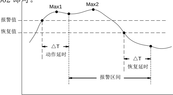
上限报警输出控制过程示意图
