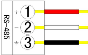
接线端子示意图
