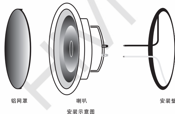
安装示意图
