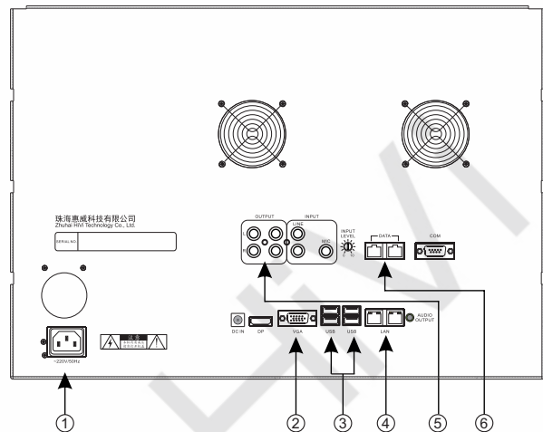
后面板
