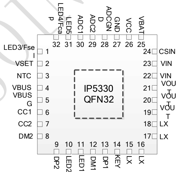
图 2 IP5330 引脚图
