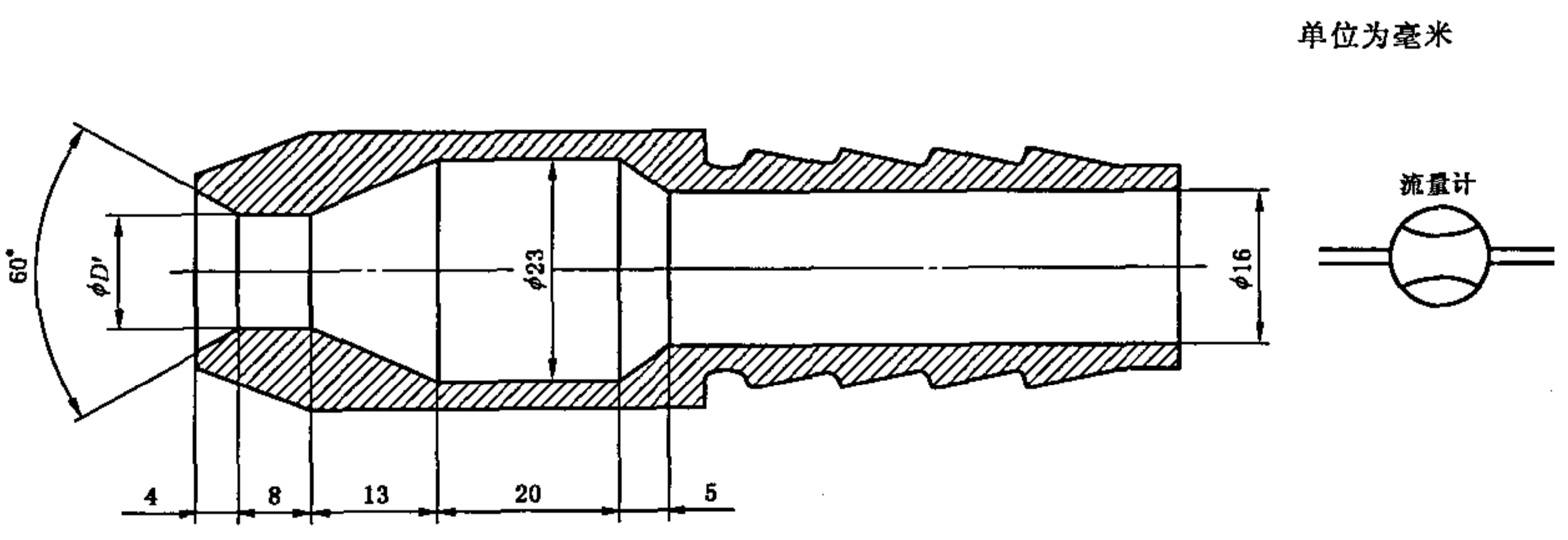
图 D.4 标准的喷水法(软管法)试验滴嘴
