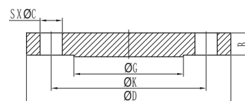
Blank Flange
