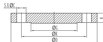
Blank Flange
