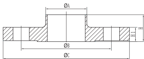
DIN 2576-DIN 11850
