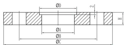
DIN 2576-DIN 11850
