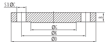
Blank Flange
