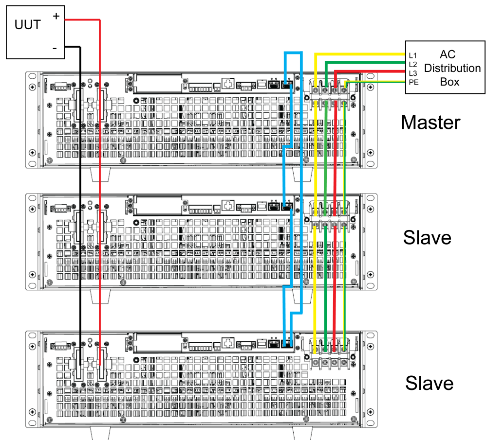
图 5-1 线路连接图
