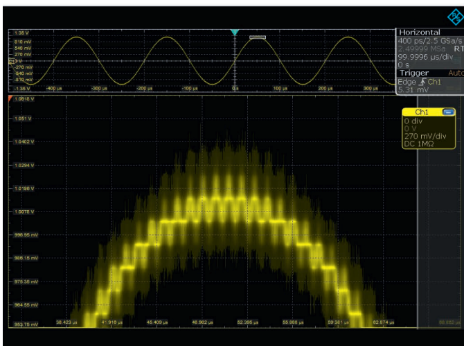
放大后的正弦波峰：未激活高分辨率模式。在缩放窗口中只能看到量化电平。
