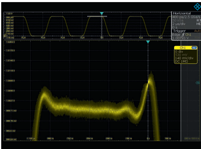
罗德与施瓦茨数字触发系统具有高灵敏度，可在低于 9 mV 的信号过冲上触发，如下图所示。在 140 mV/div 的垂直刻度下，该信号幅度只相当于一个显示刻度的一小部分。
