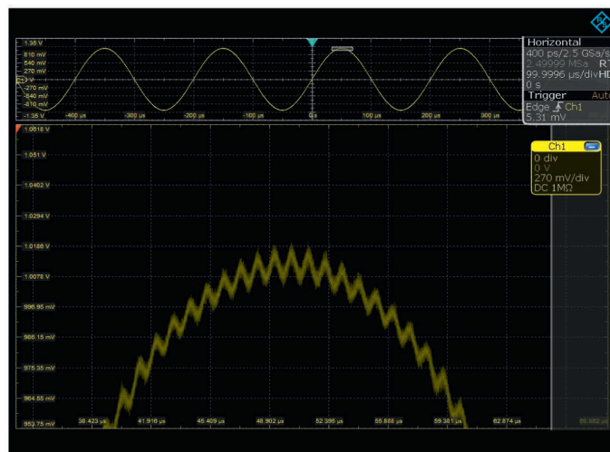
打开高分辨率模式后，缩放窗口显示出另一个幅度很低的正弦波叠加在信号上。
