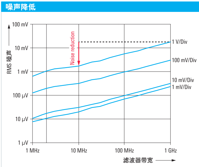
R&S®RTE110x 示波器（1 GHz 型号）的噪声与高分辨率模式下的设定滤波器带宽相关。降低噪声会提高信噪比，从而提高分辨率。
