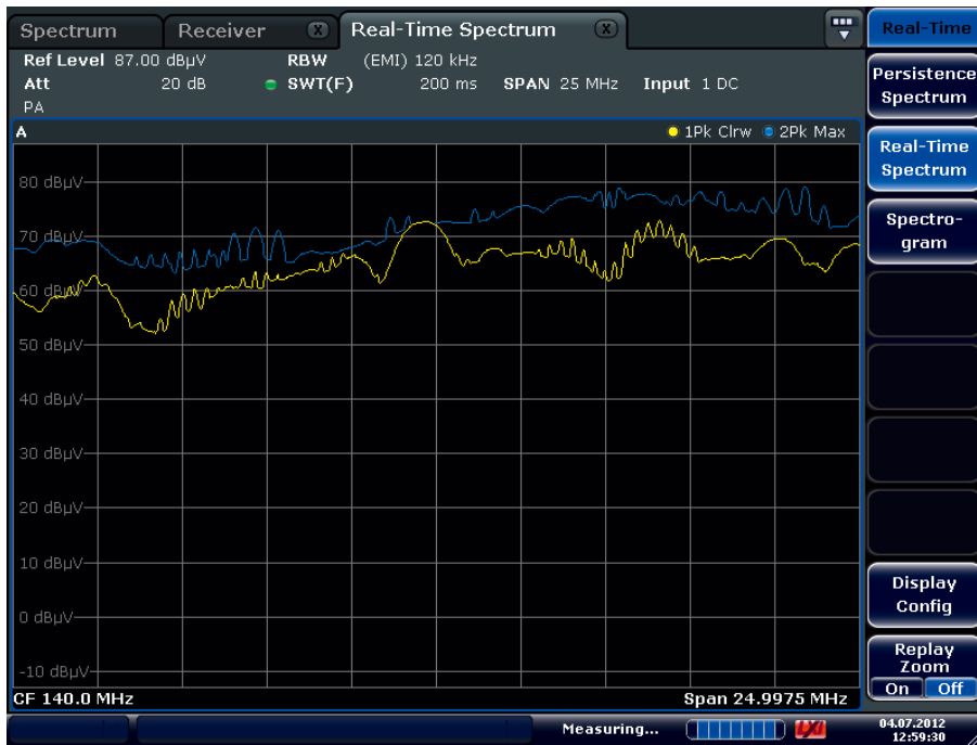
在常规分析仪模式中的宽带干扰 (本例中是由EMI抑制较差的电动机引起的) 显示。黄色轨迹代表当前的频谱，蓝色轨迹为最大值保持 (Max Hold)。
