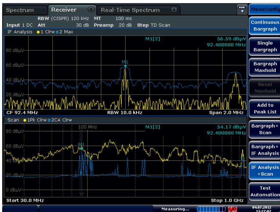
屏幕上方：使用中频分析功能，在当前EMI接收频率附近射频输入信号的连续频谱显示。 屏幕下方：预览测量的保存结果。上图中的中心频率由下图中的标记位置控制(标记跟踪功能)。或者，中频频谱显示的数值和柱状图三者可以联动。
