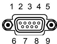
BT3562 (9 针) 连接器
