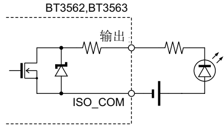
与 LED 的连接
