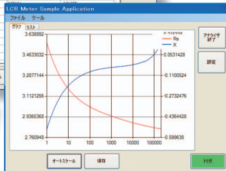
LCR标配软件所显示的扫频测量结果的明细图表界面
