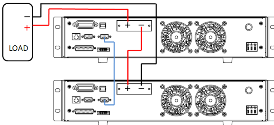
图 1 两台串联的电源设备示意图
