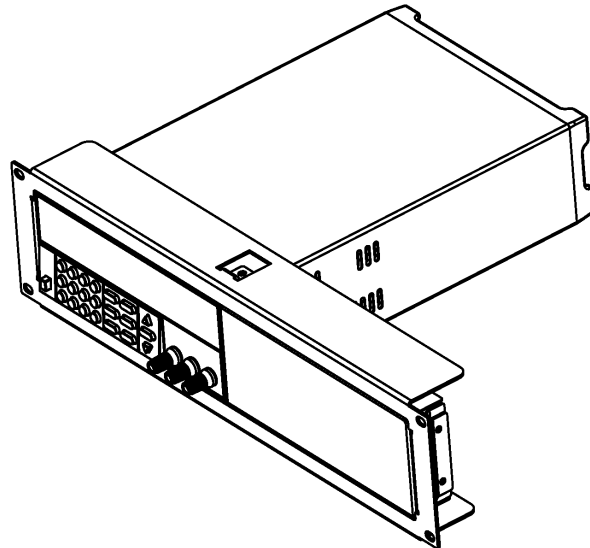
图 1.2 单个仪器上架安装的侧视图
