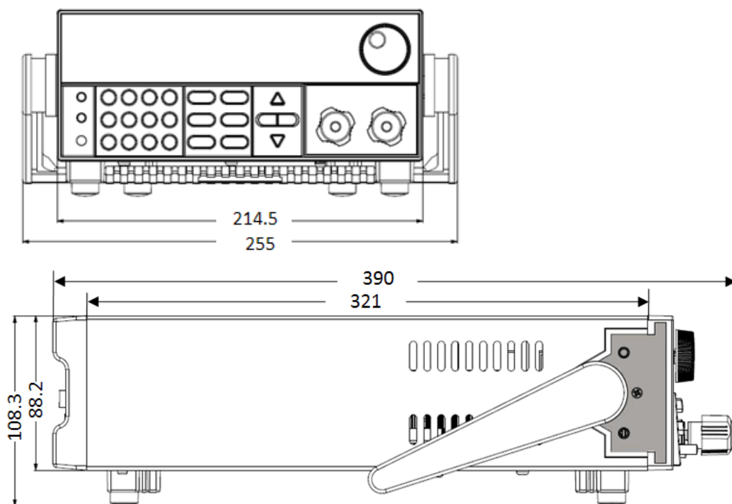
详细尺寸图
