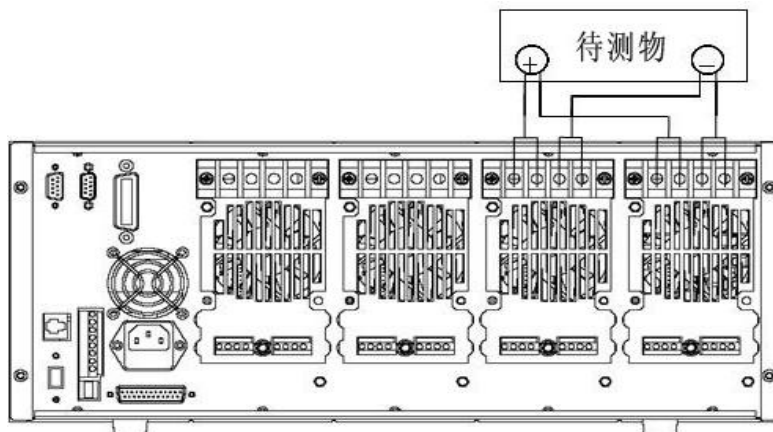
图 3-12 负载并联连接图
