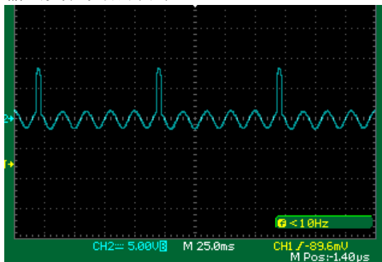
突波波形
