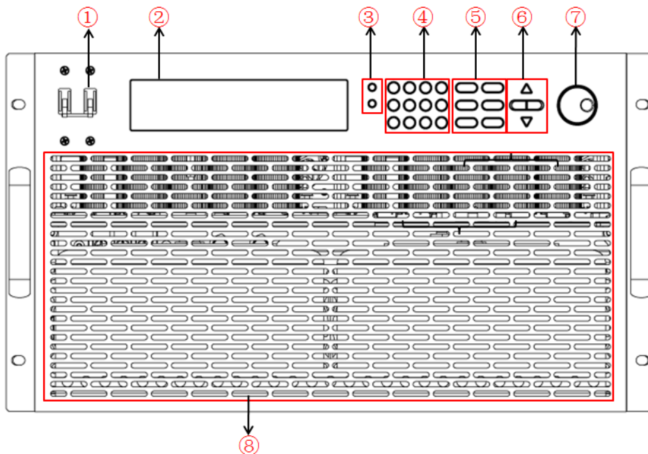
IT7326H 前面板
