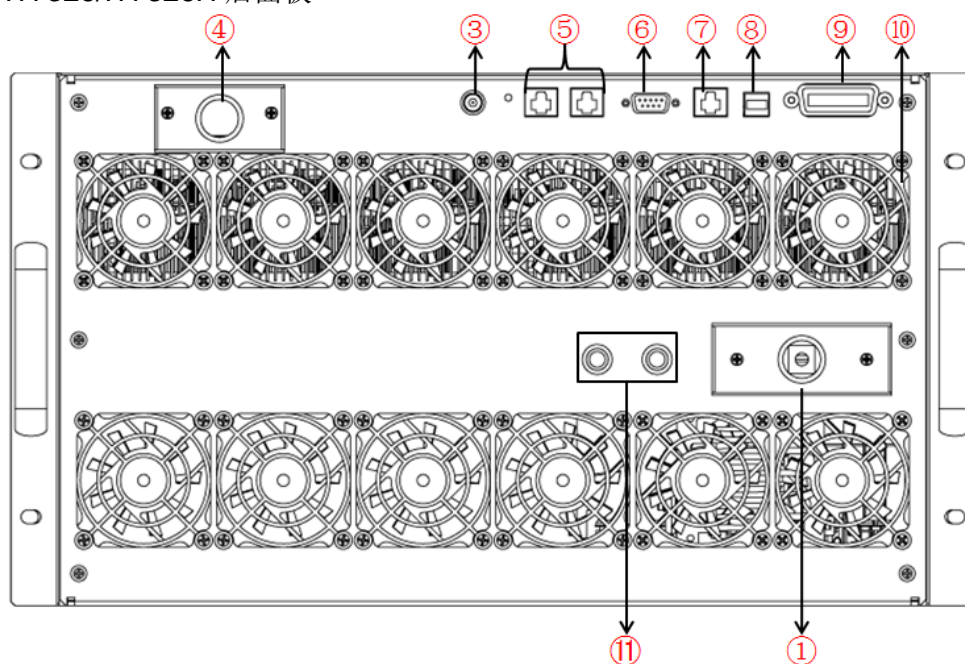
IT7326/IT7326H 后面板
