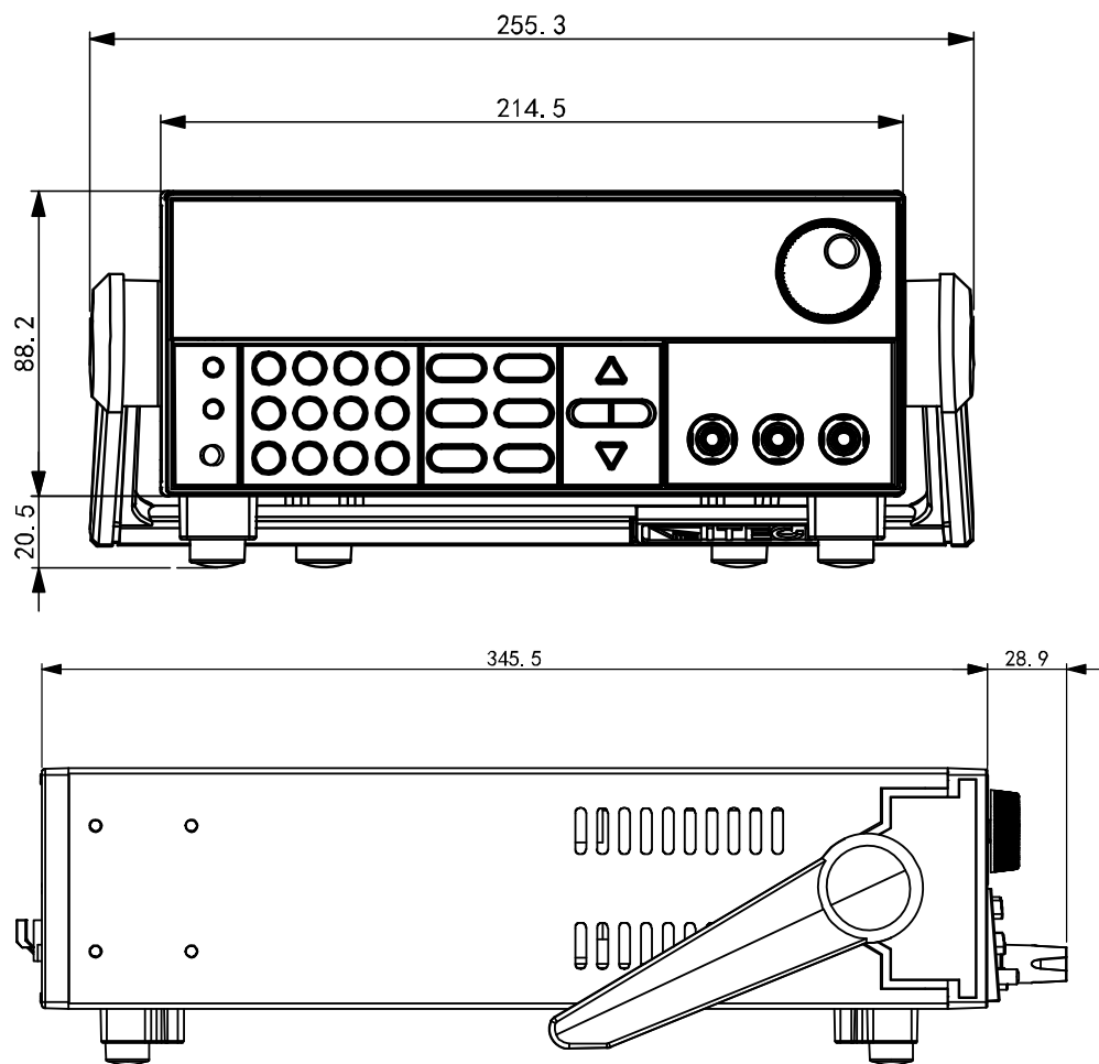
详细尺寸图
