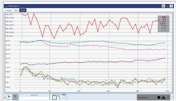
数据记录器多通道示图显示屏幕。
