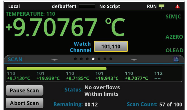
使用 DAQ6510 扫描状态屏幕，迅速简便地监测测试状态。
