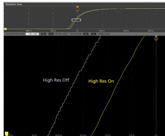
5 系列 MSO 的 12 位 ADC 与全新 High Res 模式相结合, 实现了业界领先的垂直分辨率。
