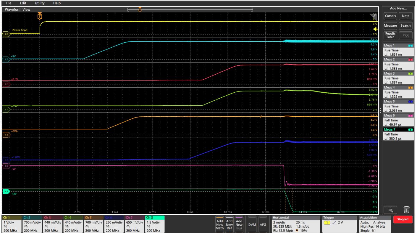
堆叠显示模式可以方便地查看所有波形，同时每个输入上保持最大 ADC 分辨率，实现最准确的测量。
