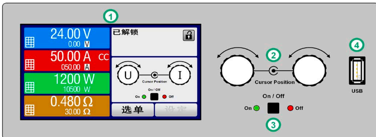
图 6 - 控制面板
