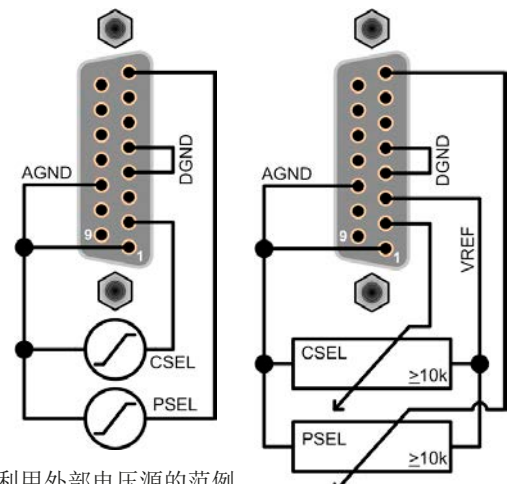
利用电位器的范围
