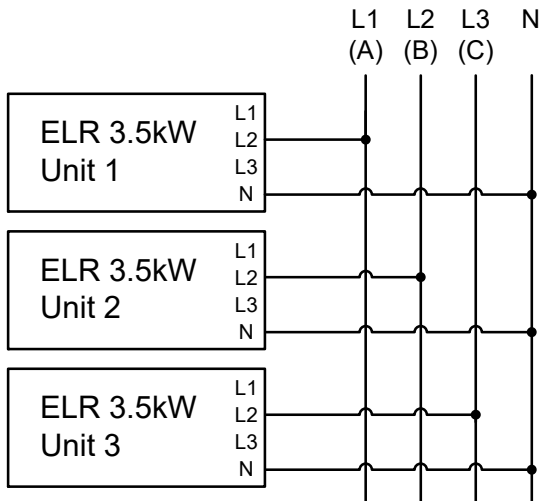
图 8 - 多台3.5 kW型号交流端连线举例
