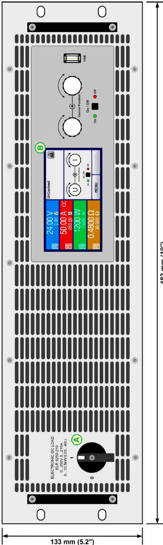
图 1 - 前视图
