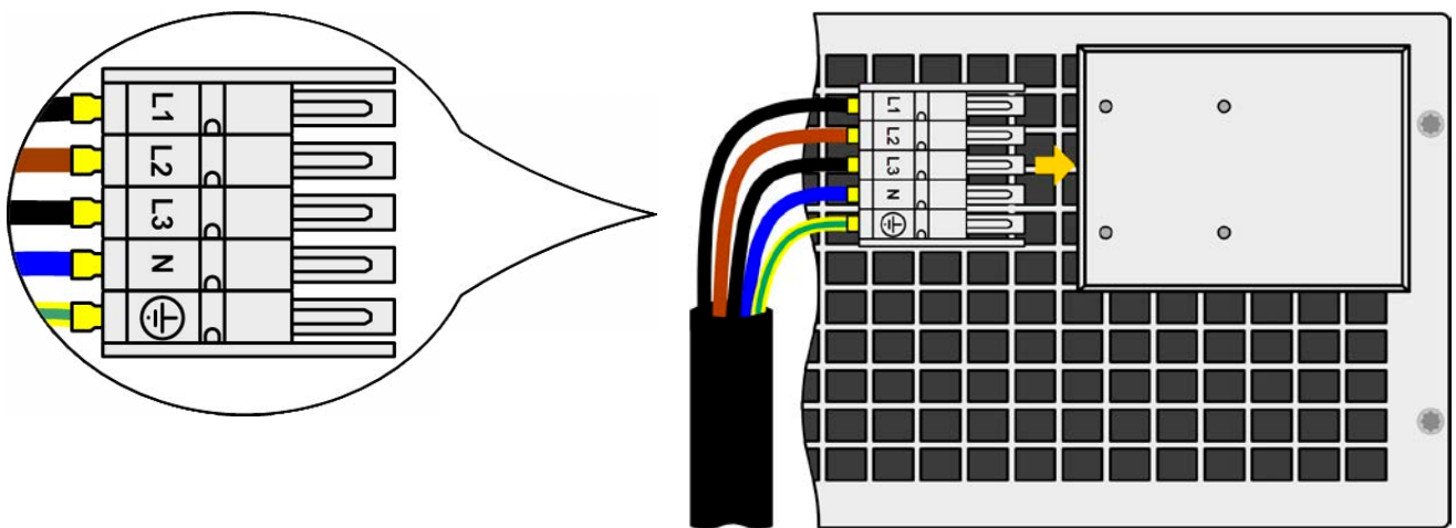
图 7 - 供电端连接线范例（随货不含此连线）
