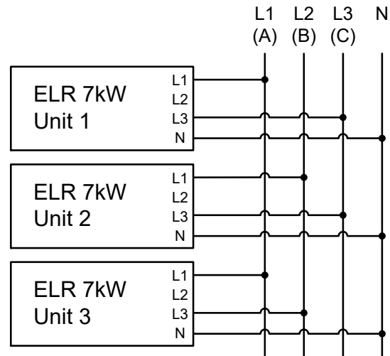
图 9 - 多台7 kW型号交流端连线举例
