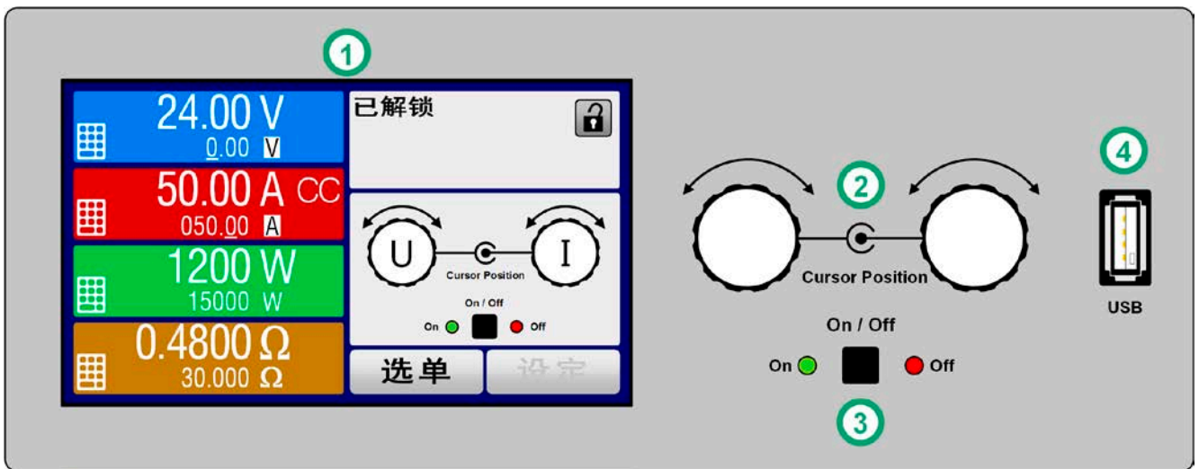
图 6 - 控制面板
