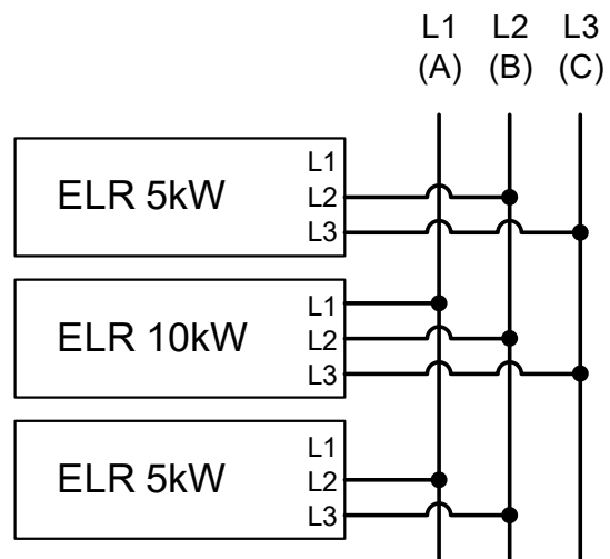
图 9 - 多台不同额定功率型号交流端连线举例，且电流基本均衡
