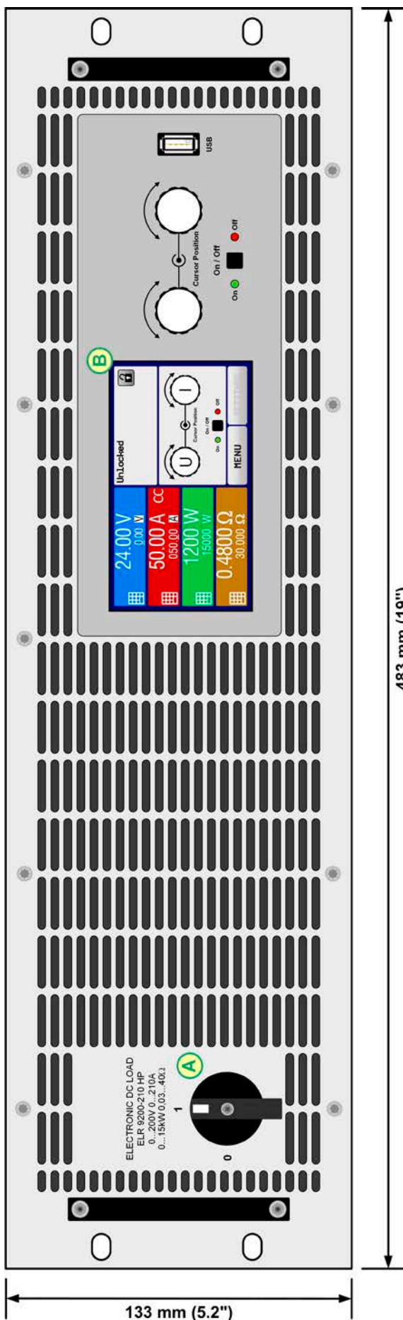
图 1 - 前视图
