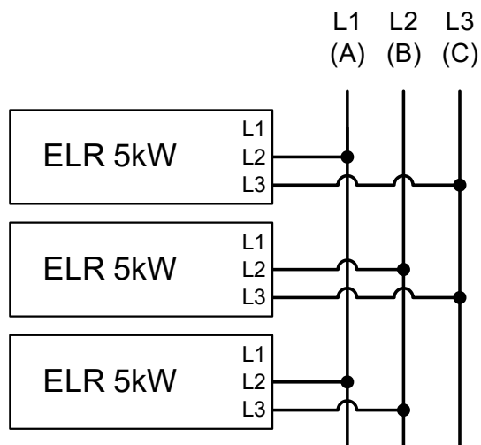
图 8 - 多台5 kW型号交流端连线举例
