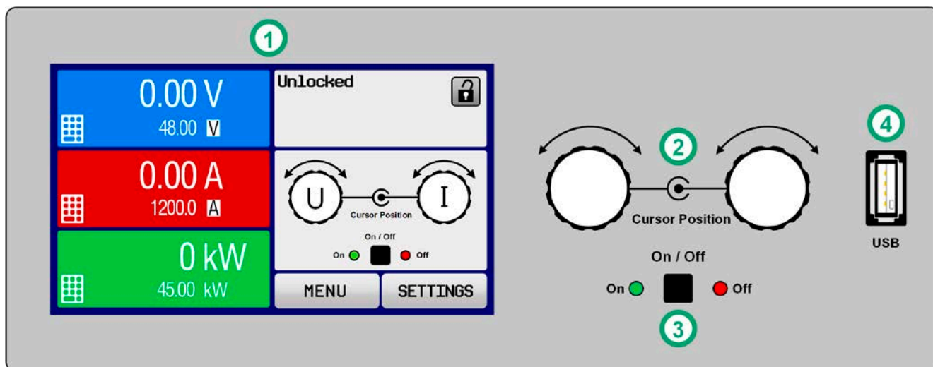
图 7 - 控制面板
