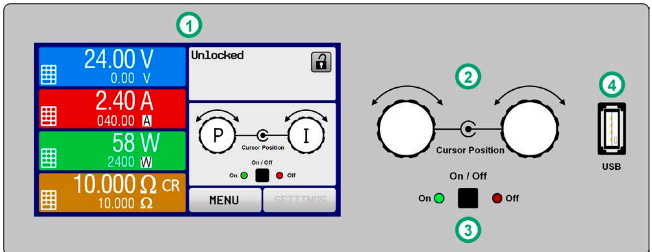
图 6 - 控制面板
