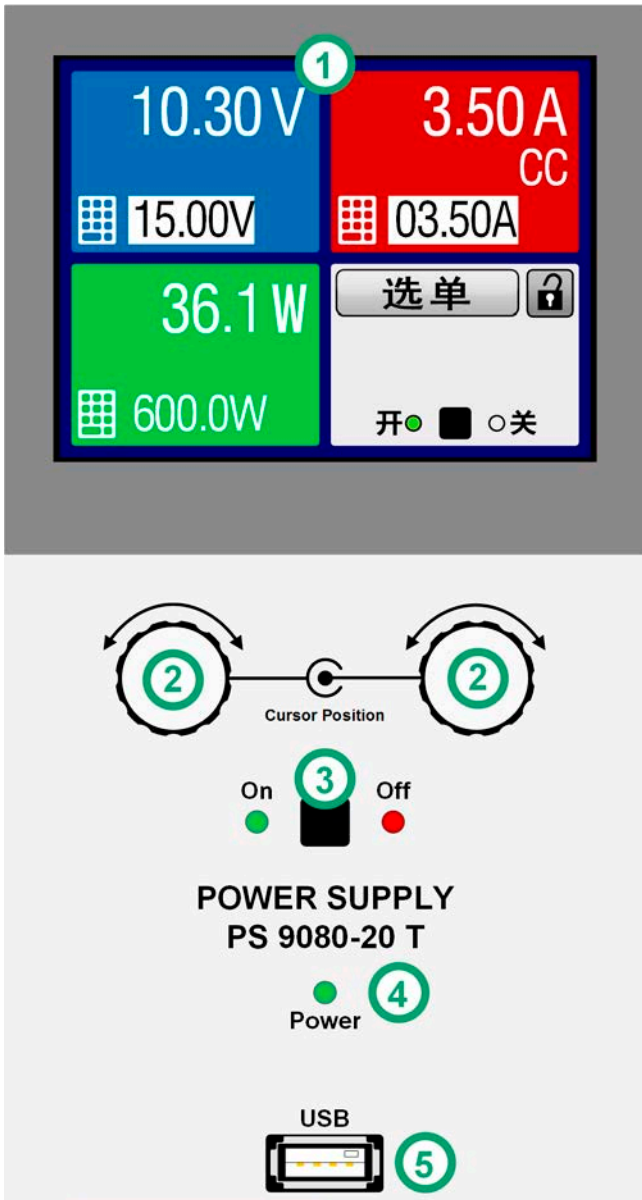
图 6 - 控制面板
