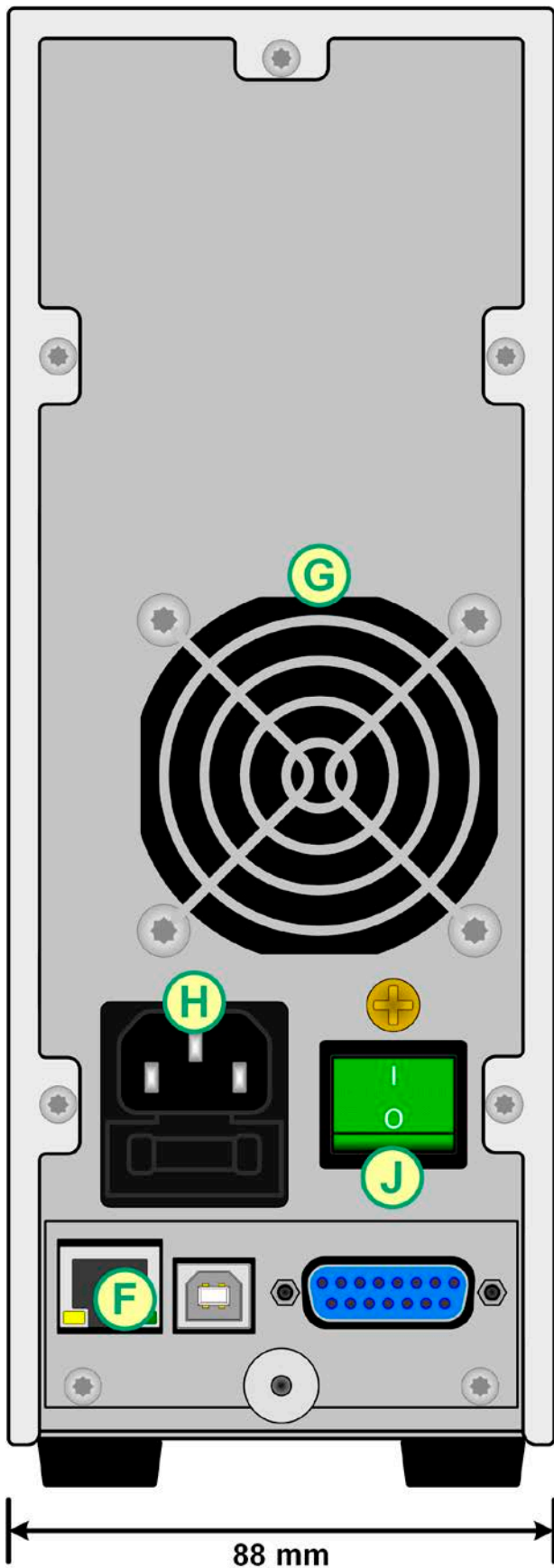
图 2 - 后视图 (显示的是320 W / 640 W型号)
