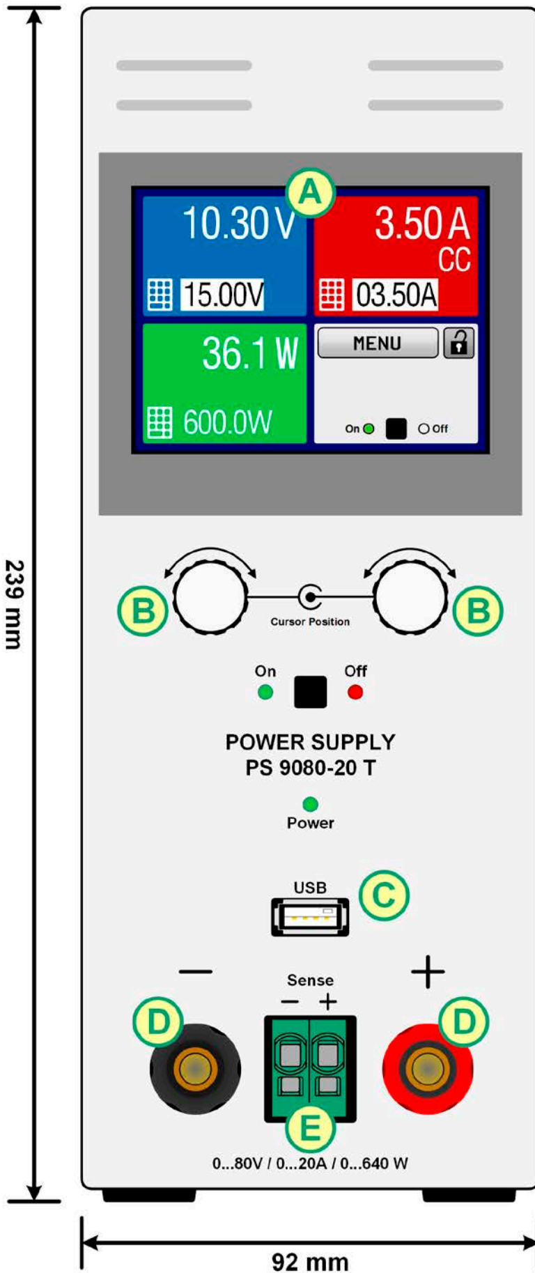
图 1 - 前视图
