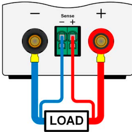
图 7- 远程感测接线原理举例
