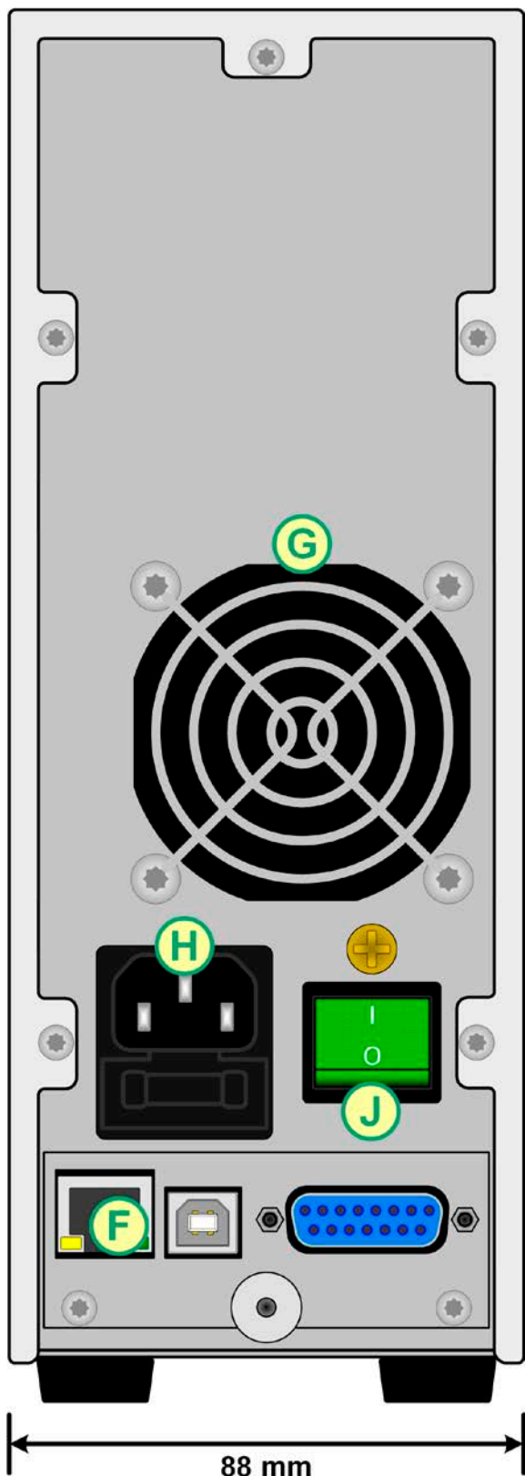
图 2 - 后视图 (显示的是320 W / 640 W型号)
