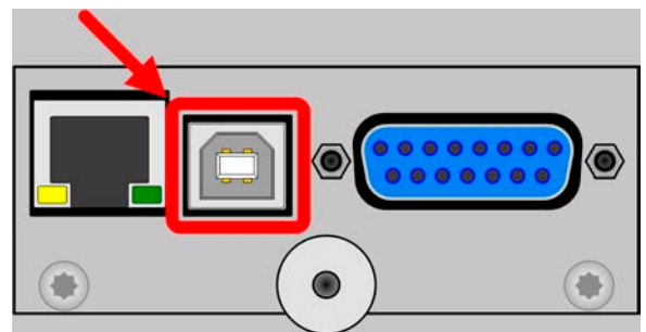
该图显示的是IF-KE4模块安装选项
