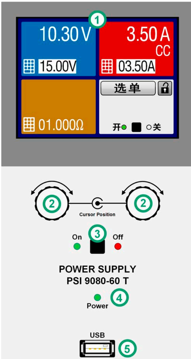
图 6 - 控制面板
