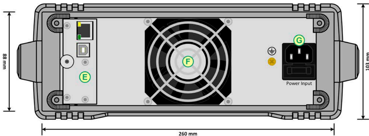
图 2 - 后视图 (所示为320W型号)
