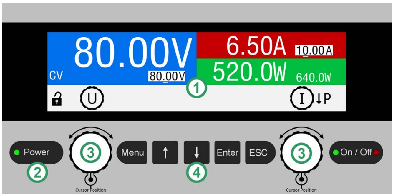
图 5 - 控制面板
