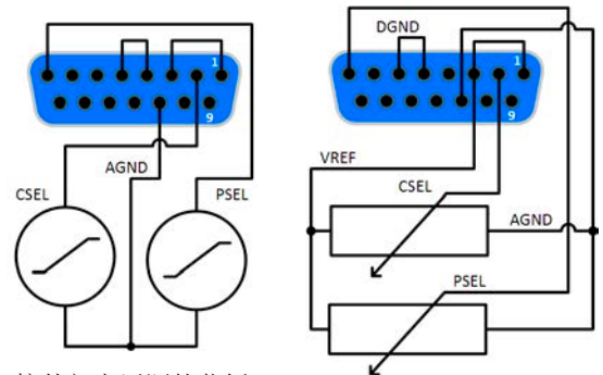
接电位器的范例
