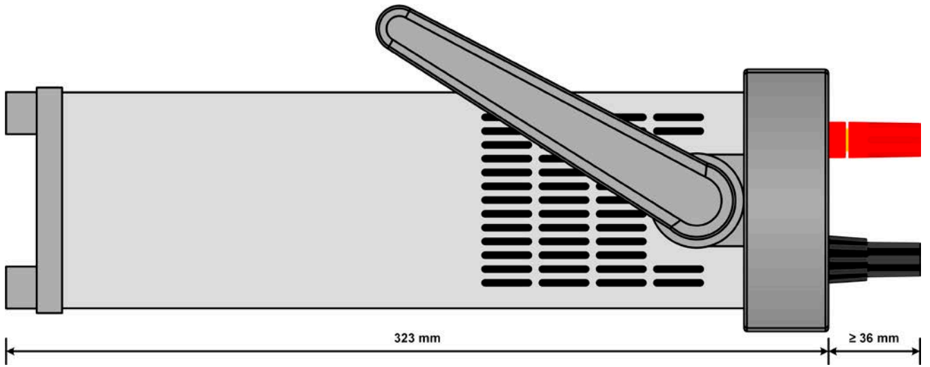
图 3 - 左侧视图，水平位（所示为320W型号）
