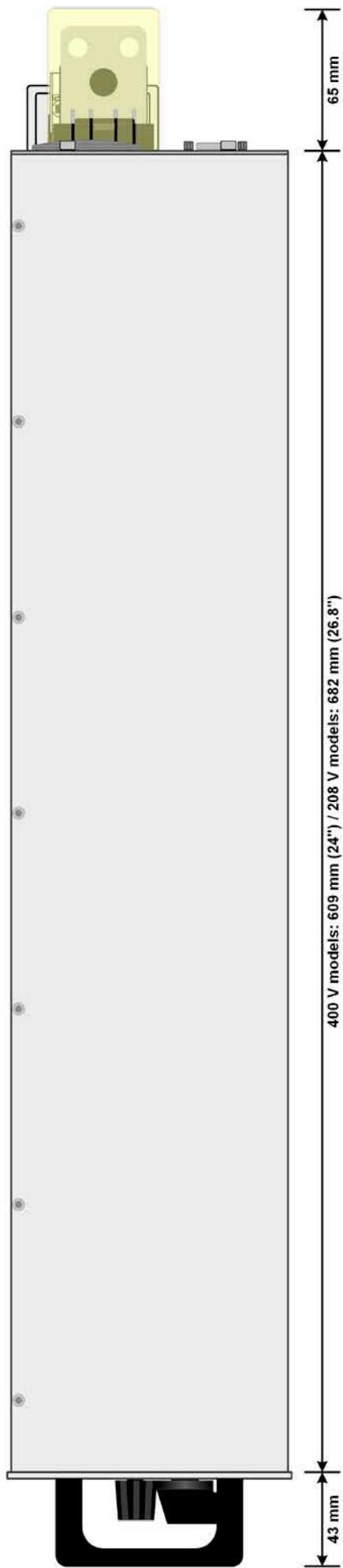
图 6 - 侧视图 (左边)
