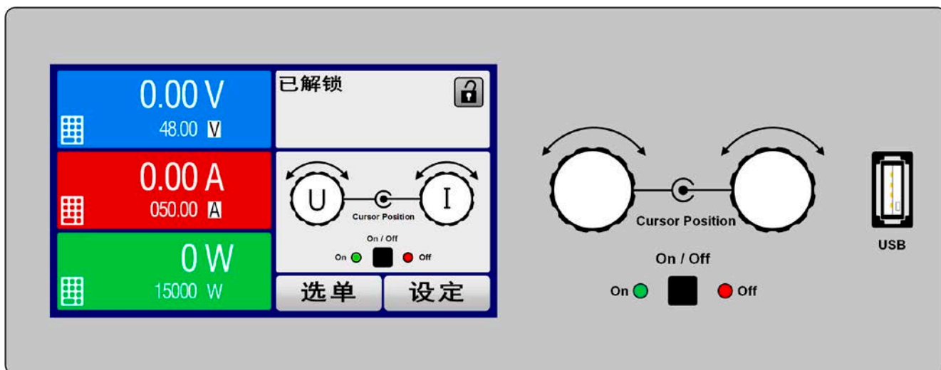
图 8 - 控制面板
