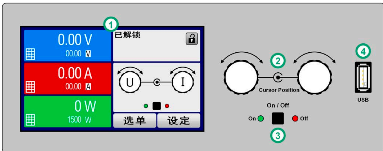
图 6 - 控制面板
