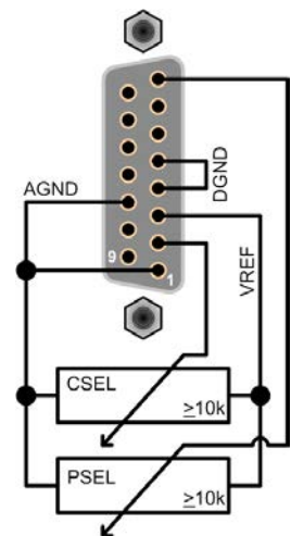
利用电位器的范例
