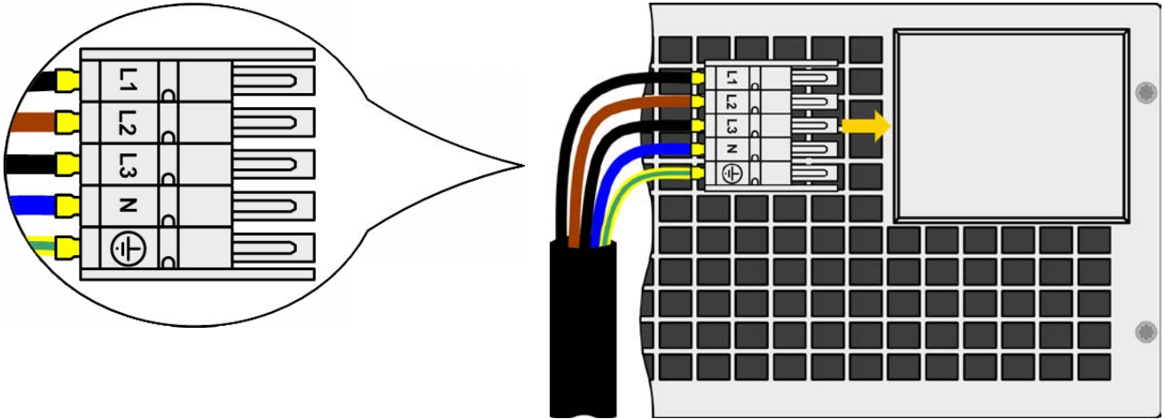
图 7 - 供电端连接线范例（随货不含此部件）
