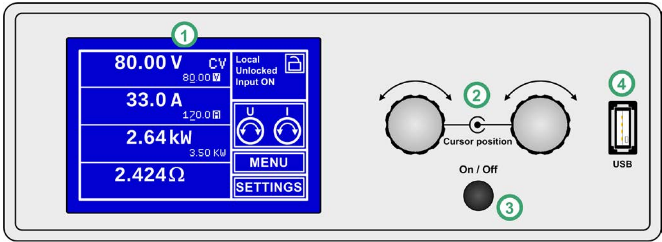
图 6 - 控制面板
