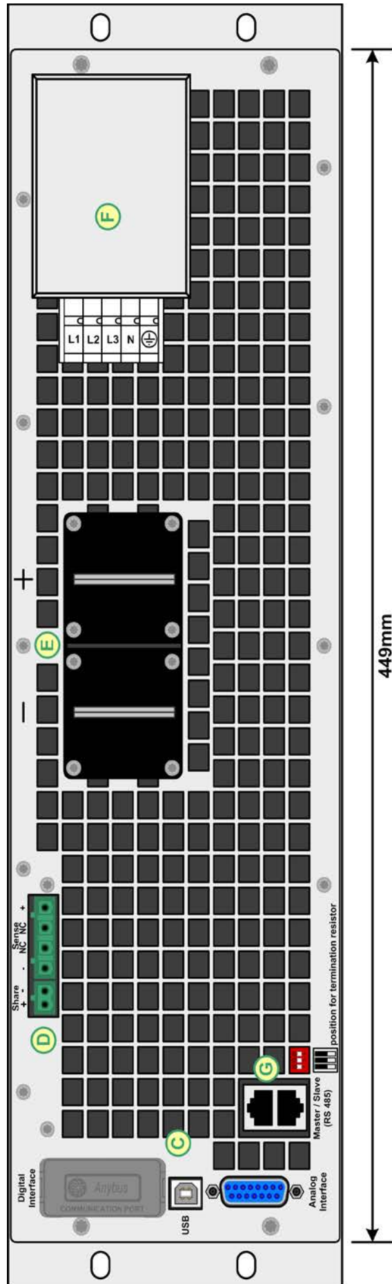
图 2 - 后视图
