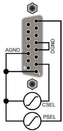
利用外部电压源的范例
