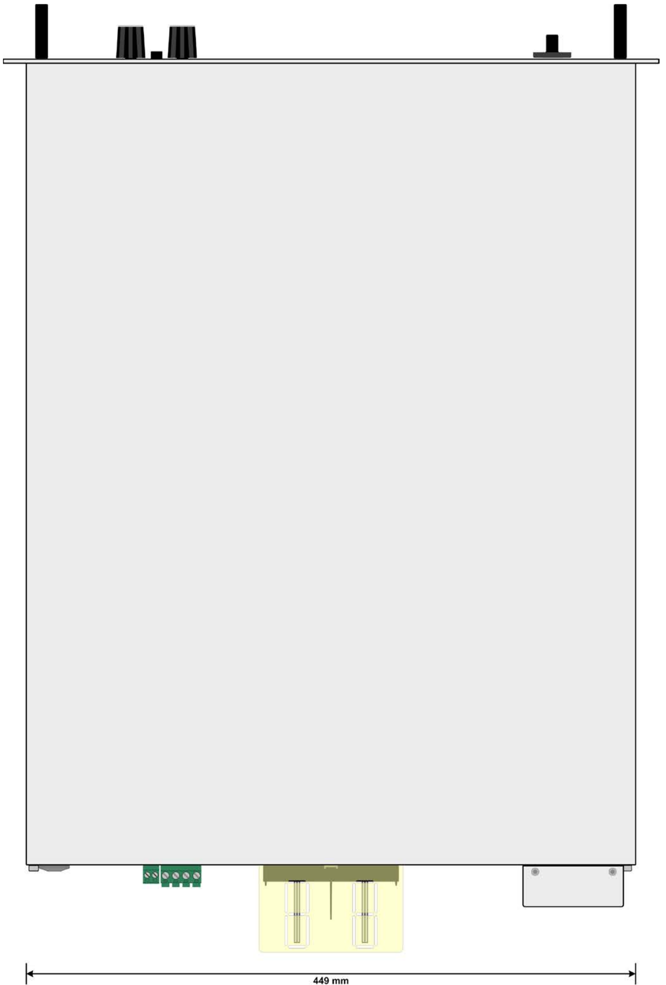
图 5 - 俯视图
