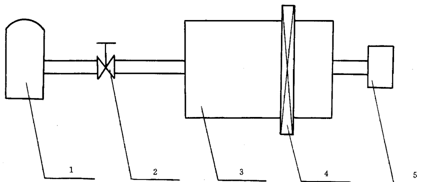
1—储气罐；2—调节阀；3—静压箱；4—被测阀；5—气量计
