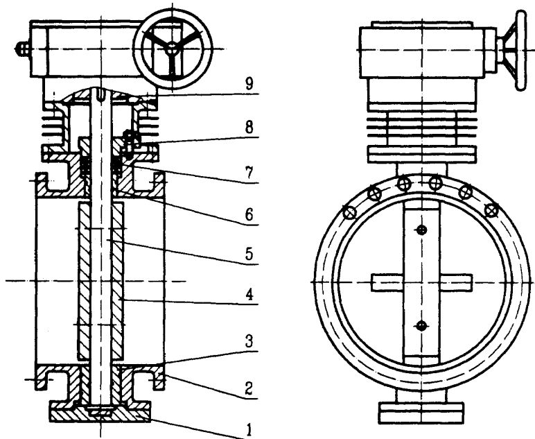
1—端盖；2—阀体；3—轴承；4—蝶板；5—阀杆； 6—毡圈；7—填料；8—填料压盖；9—驱动装置
